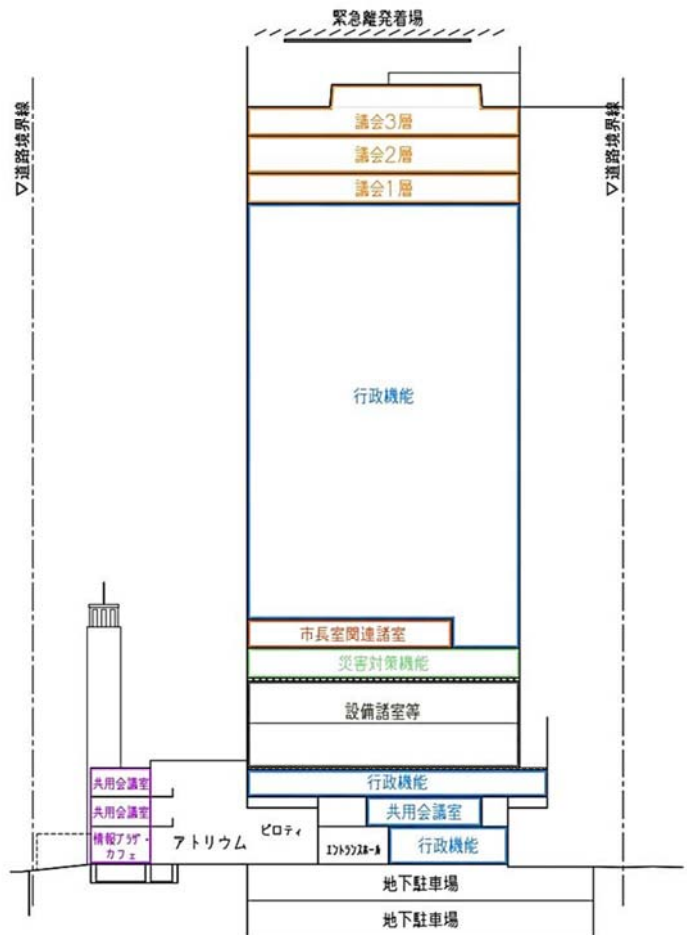
南北断面図
