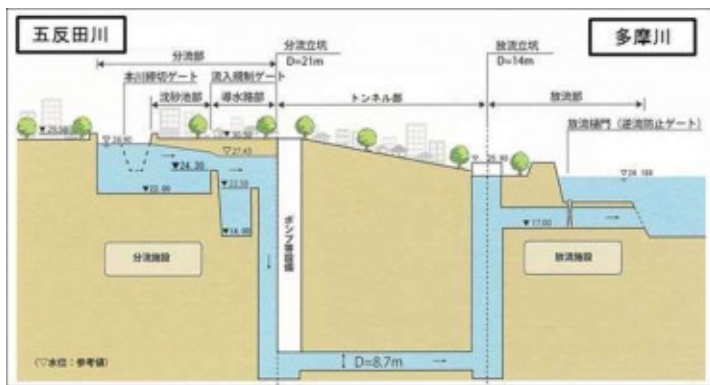
五反田川放水路の放流部完成想定図
