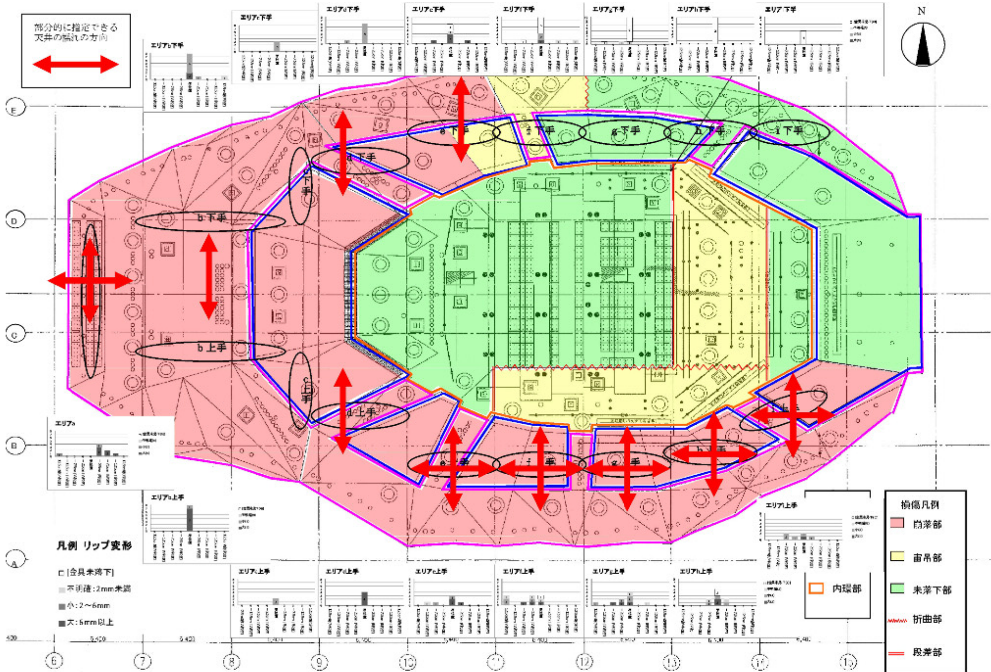
図 5.3.9 フック状金具の滑り跡及びリップ変形の分布と推定できる揺れ方向
