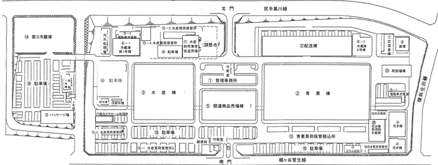
北部市場配置図
