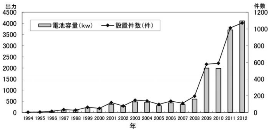
住宅用太陽光発電設備導入推移
