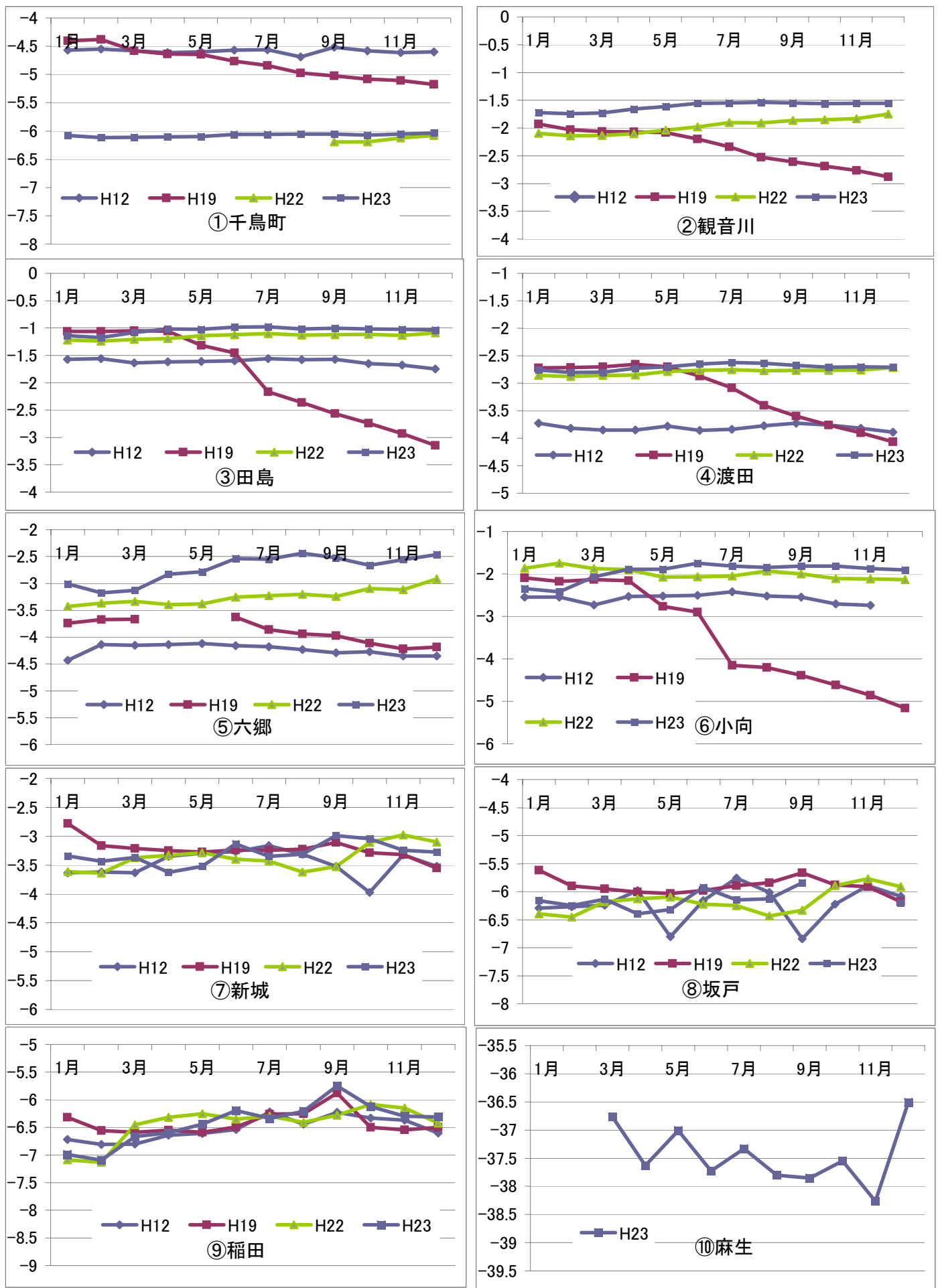
図V-12 地下水位の年間変動の経年推移（月平均・管頭から）
