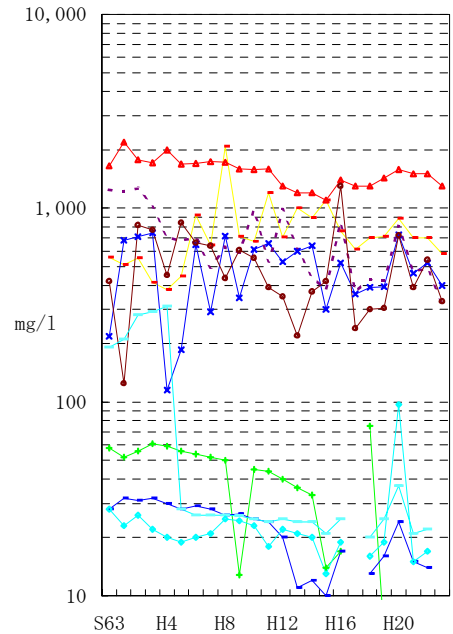
図V-16 地下水塩化物イオン濃度の経年推移
