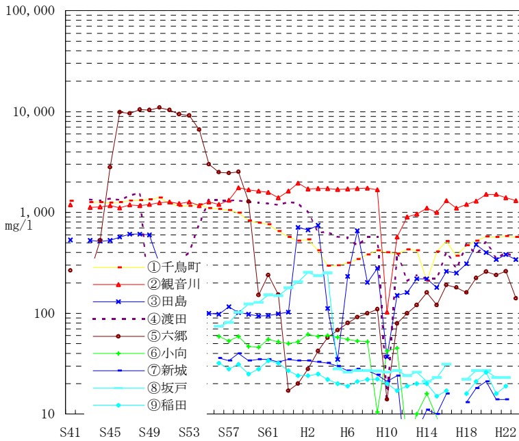
図V-16 地下水塩化物イオン濃度の経年推移
