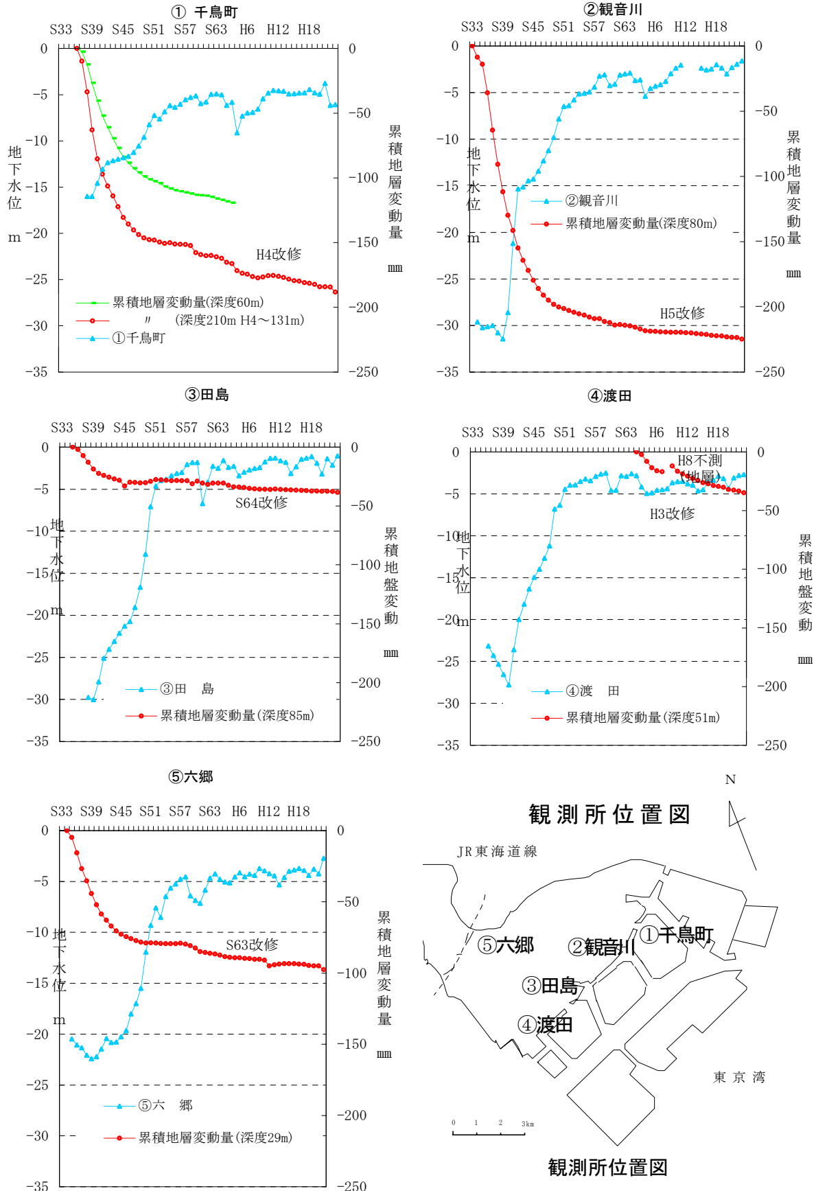
図V-15 地下水位-累積地層変動量の経年推移
