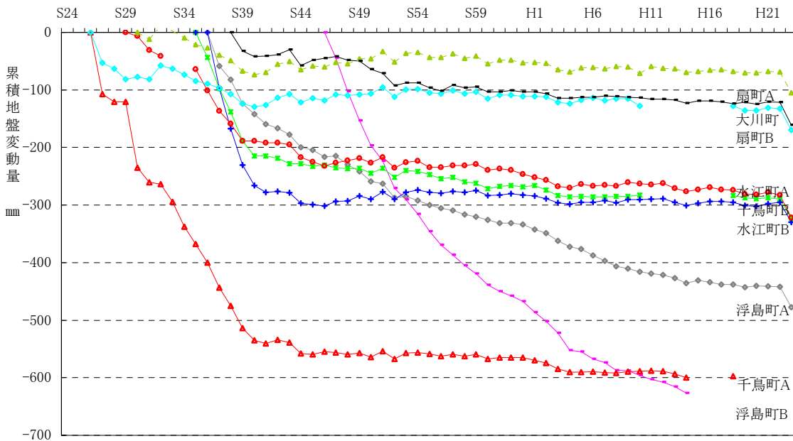
図V-8 主要水準点における累積地盤変動量の経年推移
