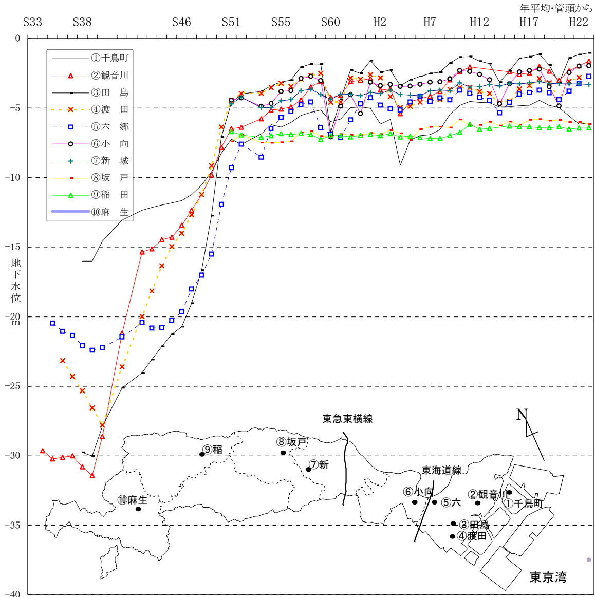
図V-13 地下水位の経年推移
