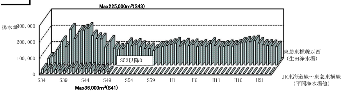
図V-3 地下水揚水量の経年推移
