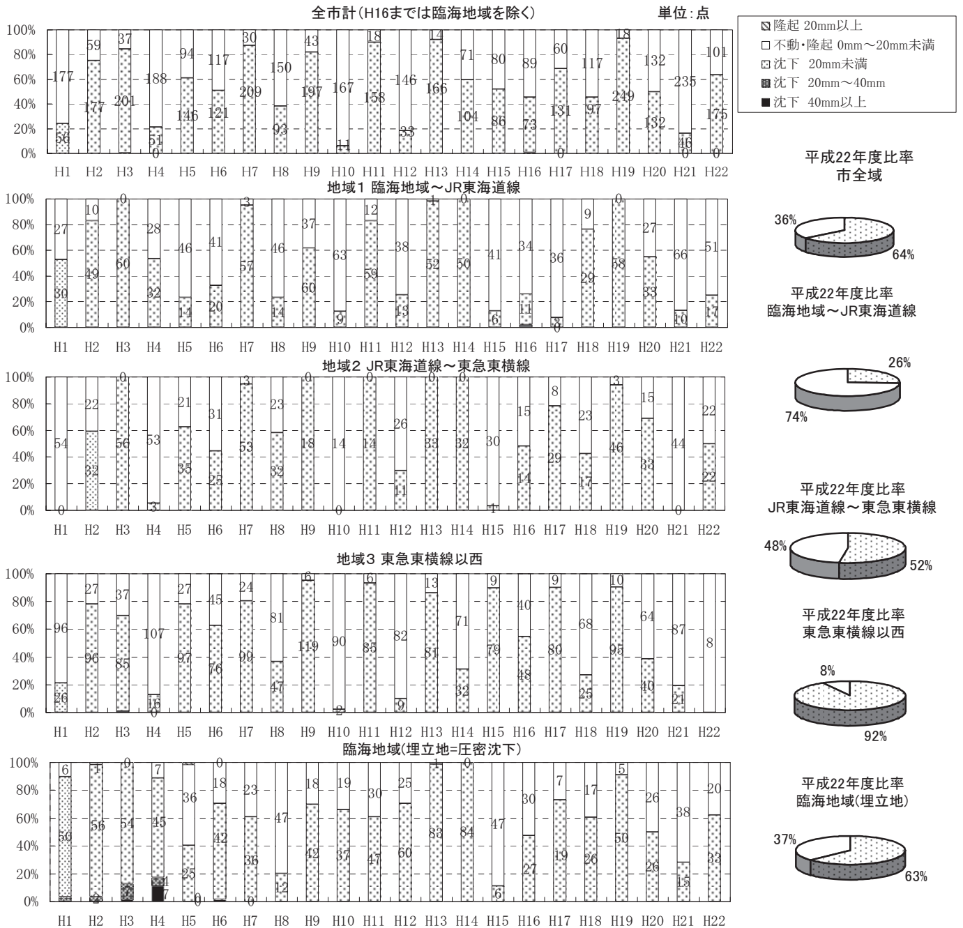
図6 精密水準測量結果の経年推移
