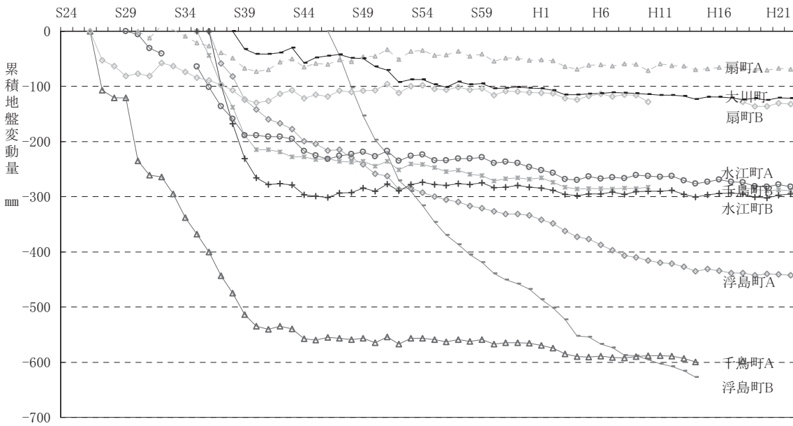
図8 主要水準点における累積地盤変動量の経年推移
