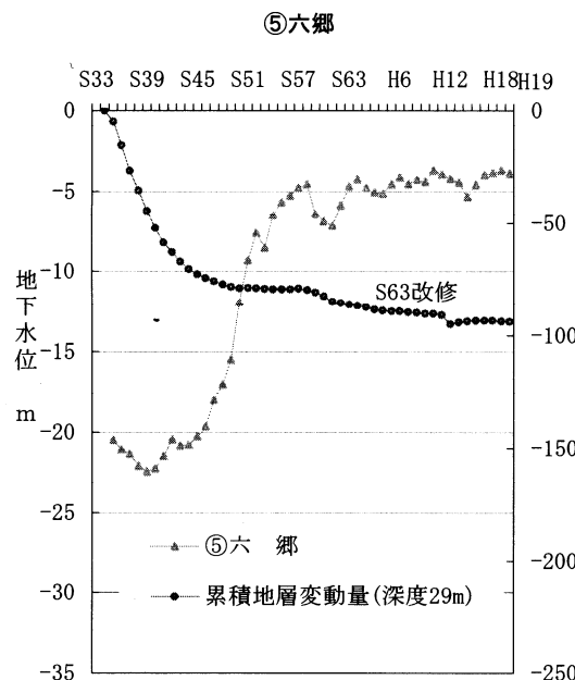
図15 地下水位-累積地層変動量の経年推移
