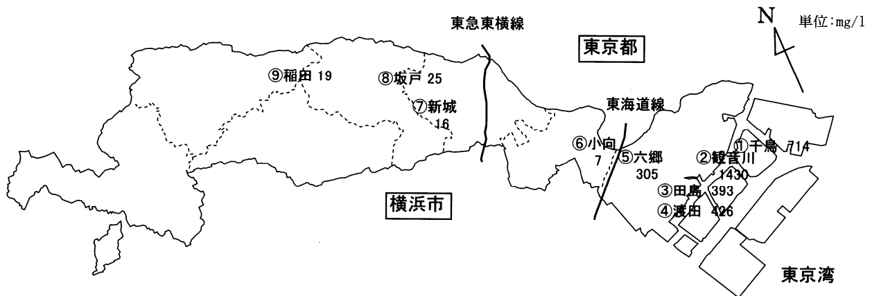
図17 地下水塩化物イオン濃度分布—下層(H19)
