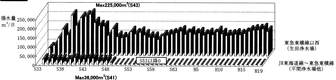
図3 地下水揚水量の経年推移
