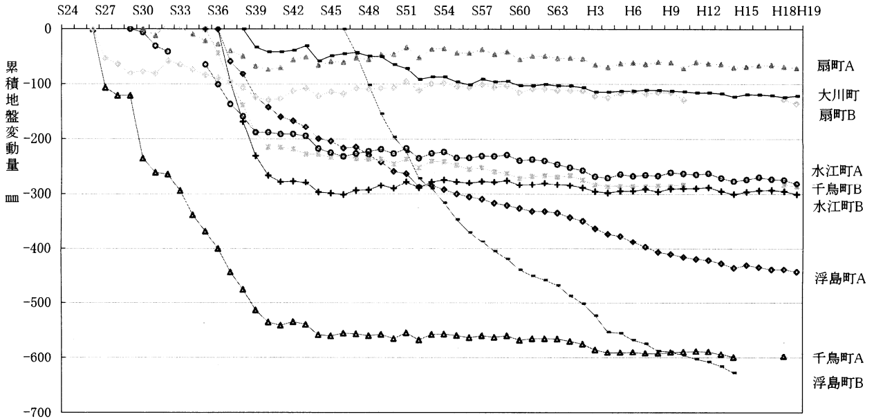
図8 主要水準点における累積地盤変動量の経年推移
