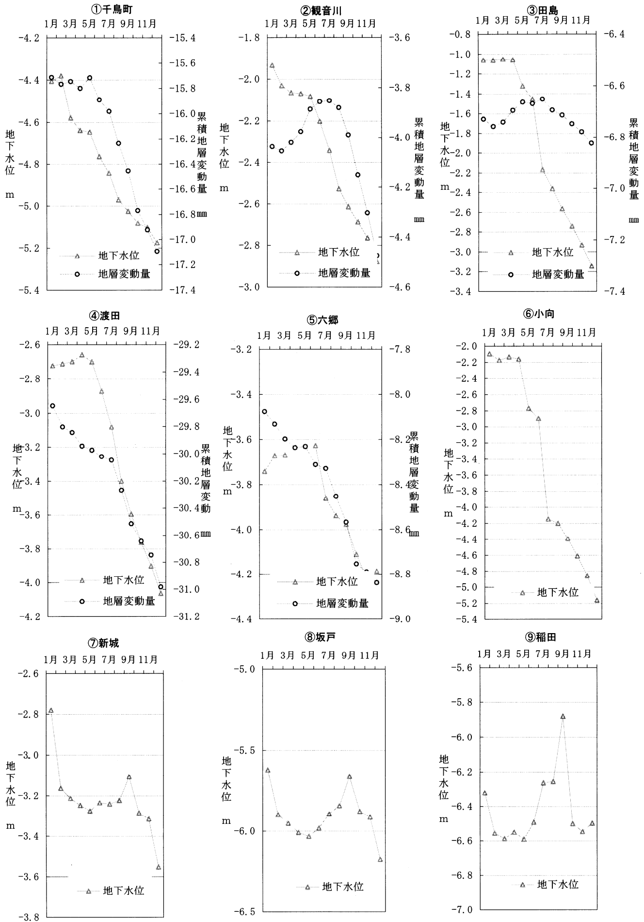
図14 地下水位-地層年間変動の年間推移 (月平均 H19.1~H19.12) (⑥~⑨は地下水位のみ)
