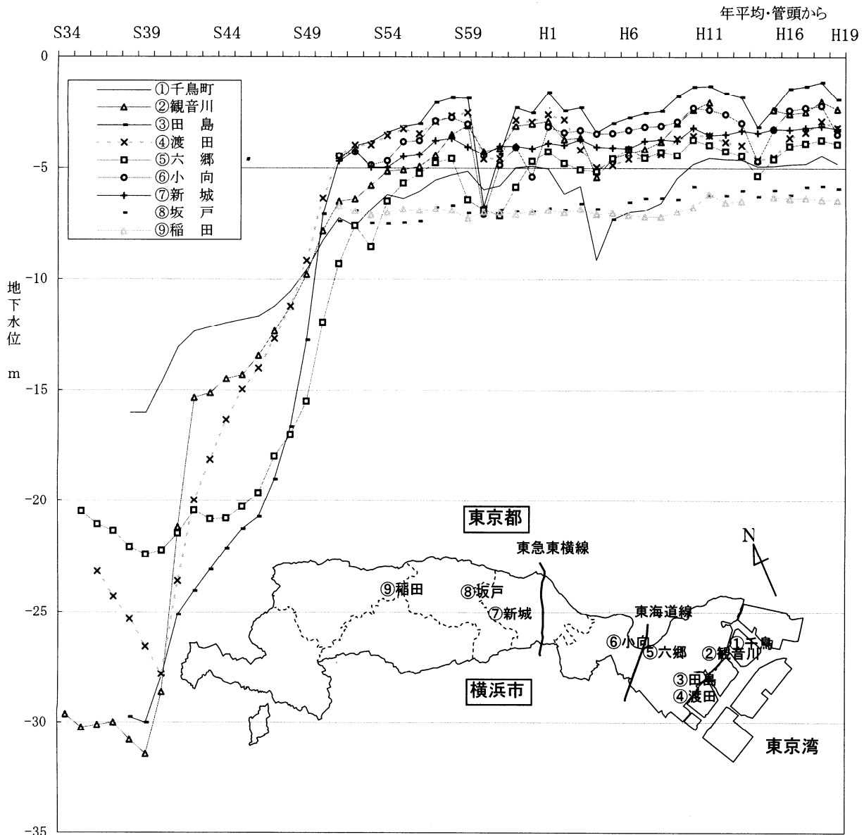
図13 地下水位の経年推移
