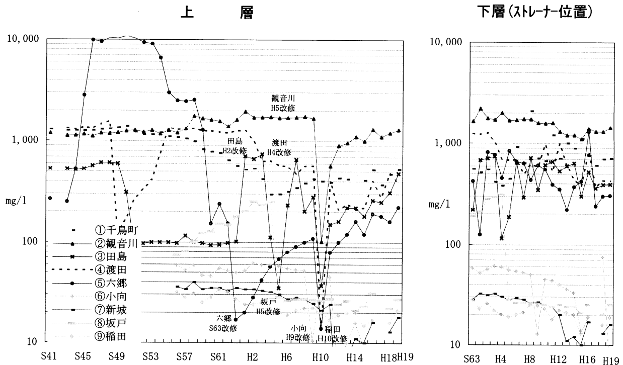
図16 地下水塩化物イオン濃度の経年推移
