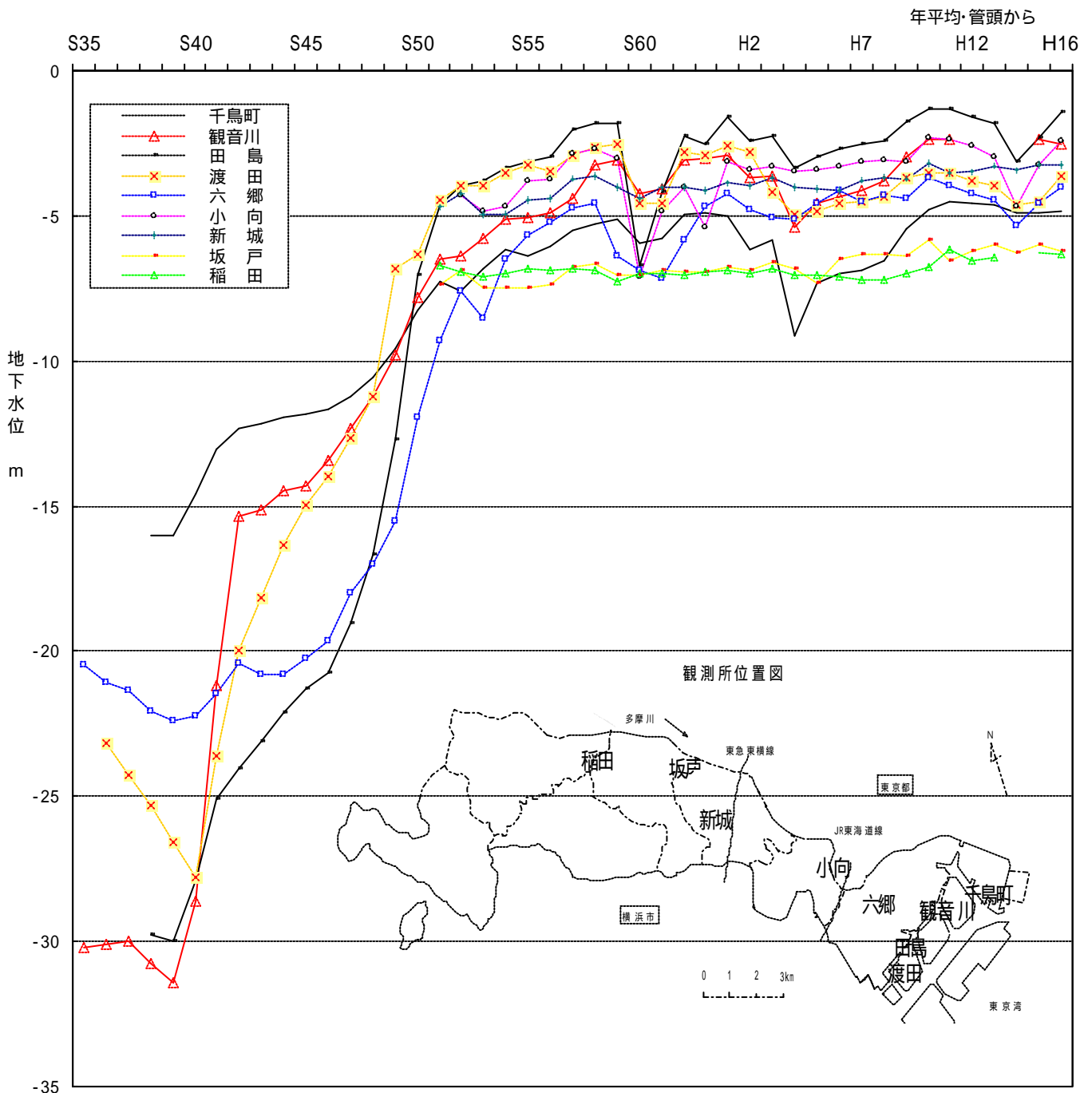
図 14 地下水位の経年推移
