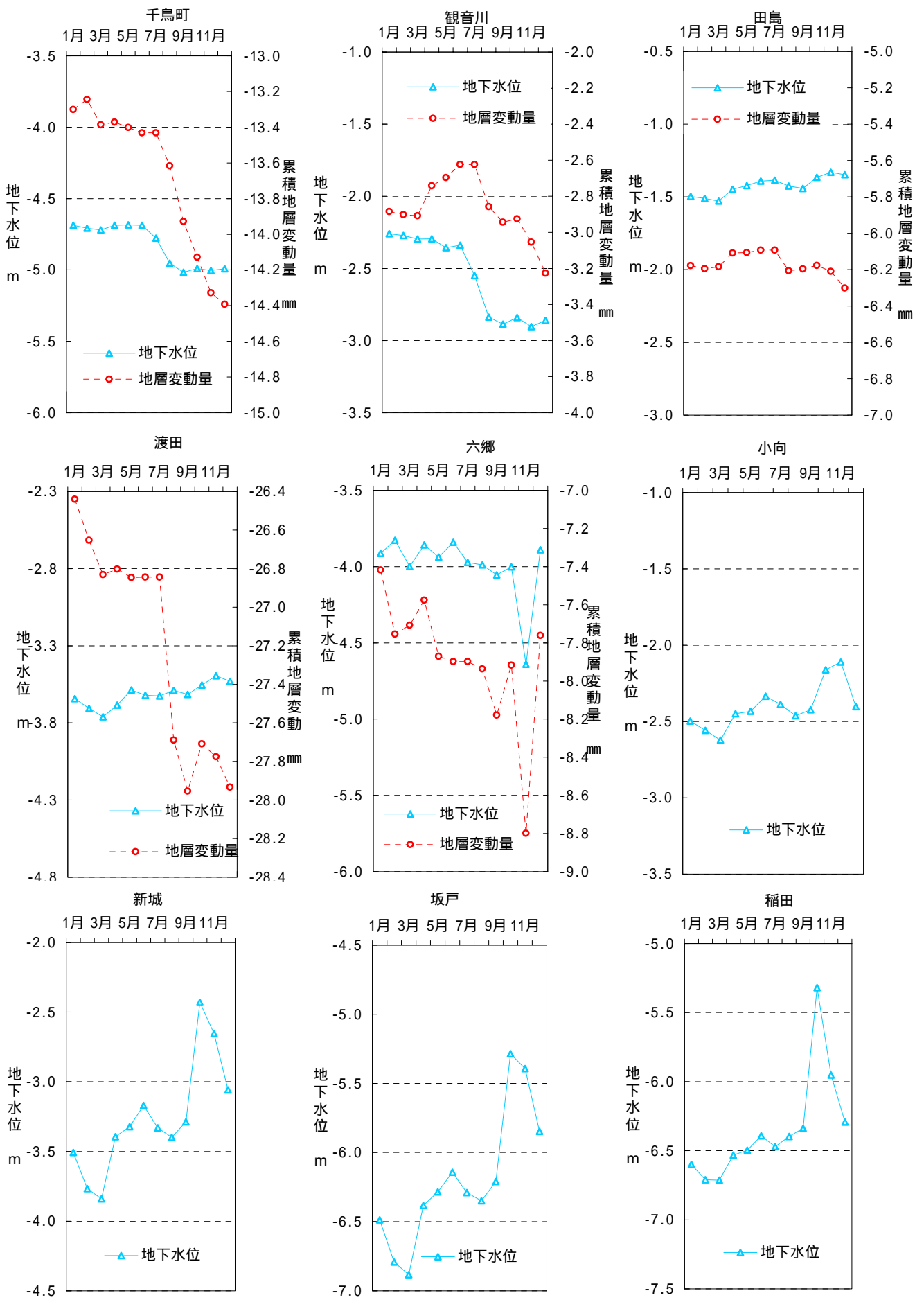
図 15 地下水水位-地層年間変動の年間推移 (月平均 H16.1~H16.12)( ~ は地下水水位のみ)
