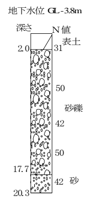
伏流水地域柱状図
