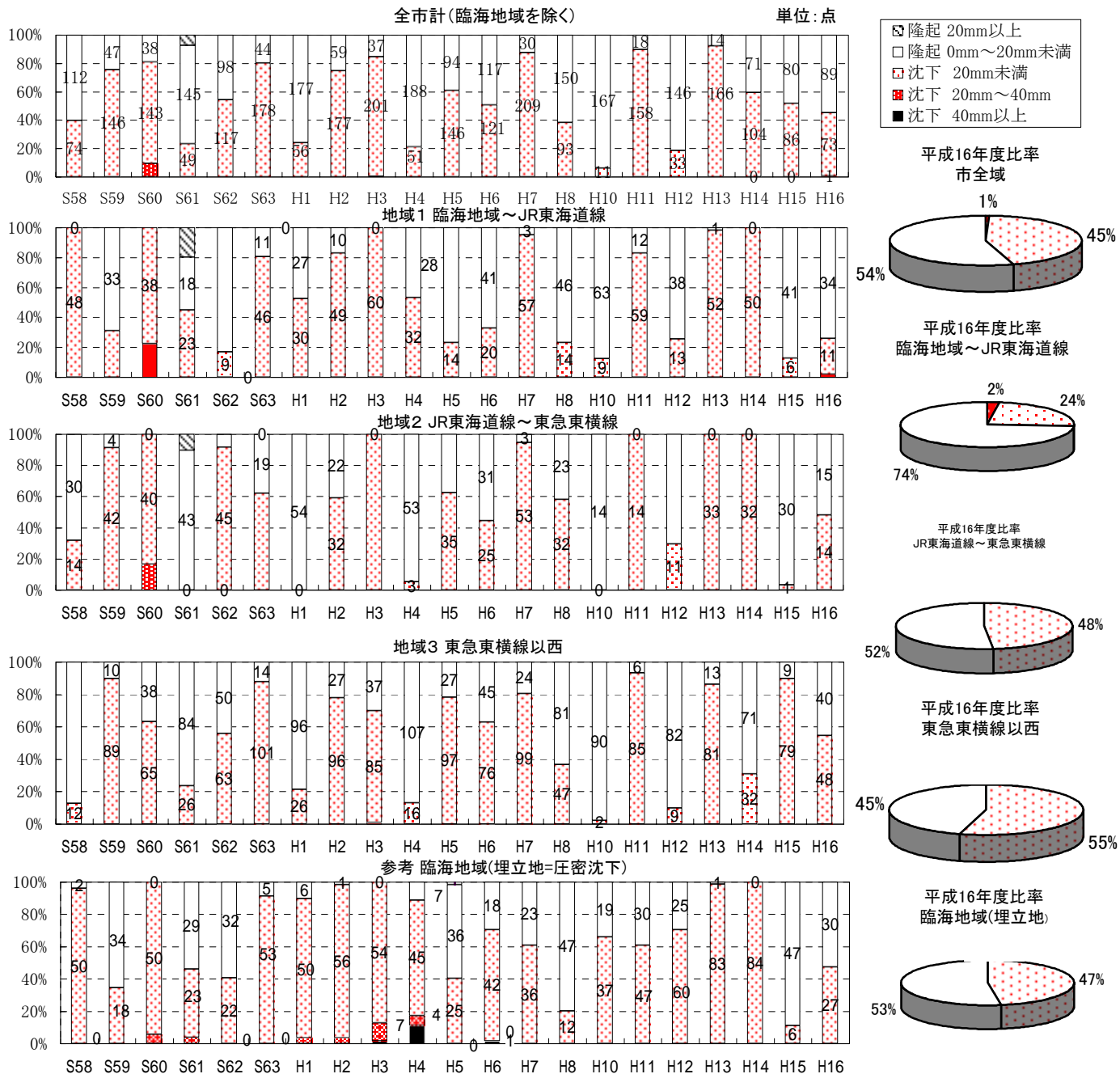
図7 精密水準測量結果の経年推移
