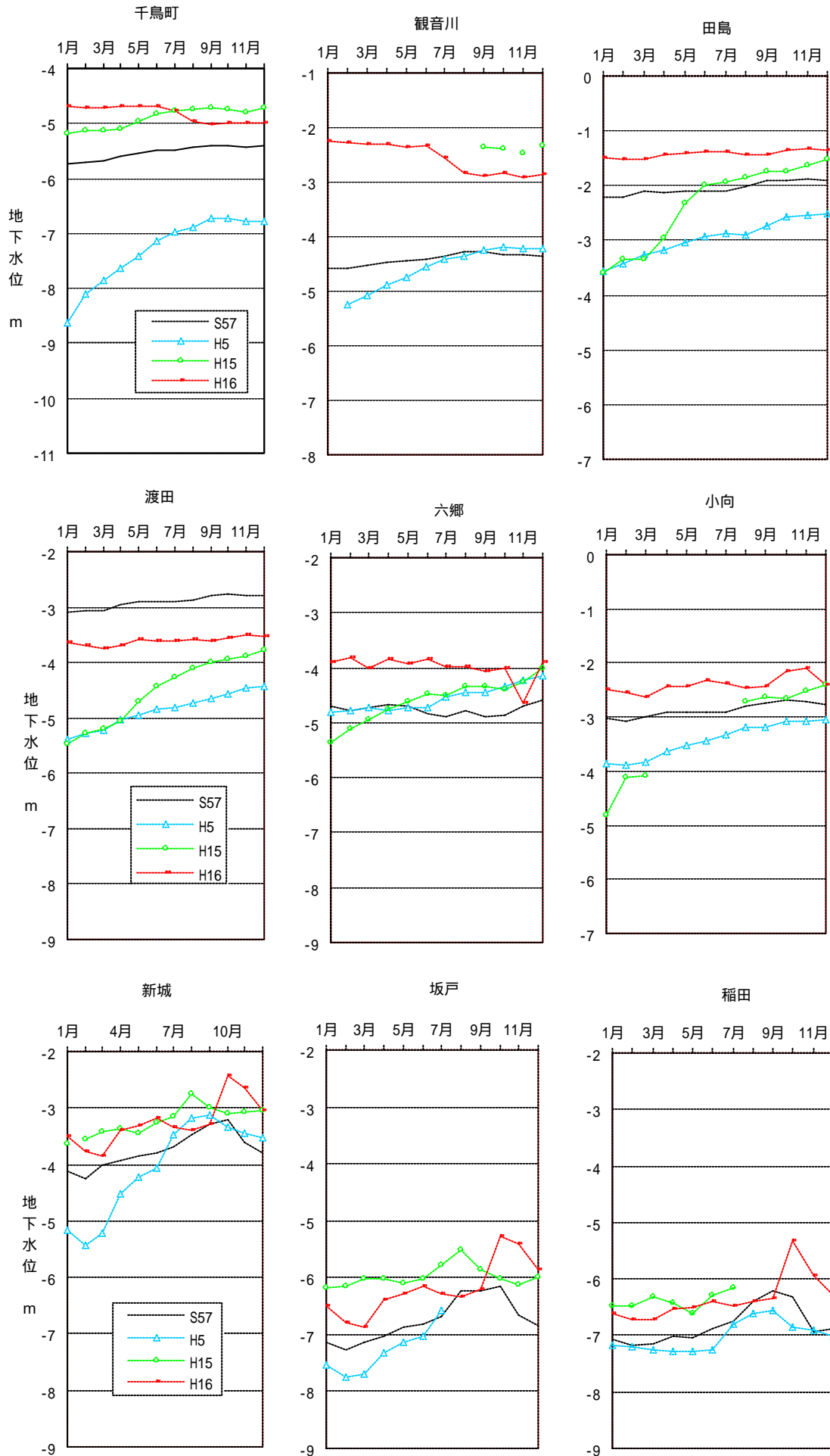
図 13 地下水位の年間変動の経年推移
