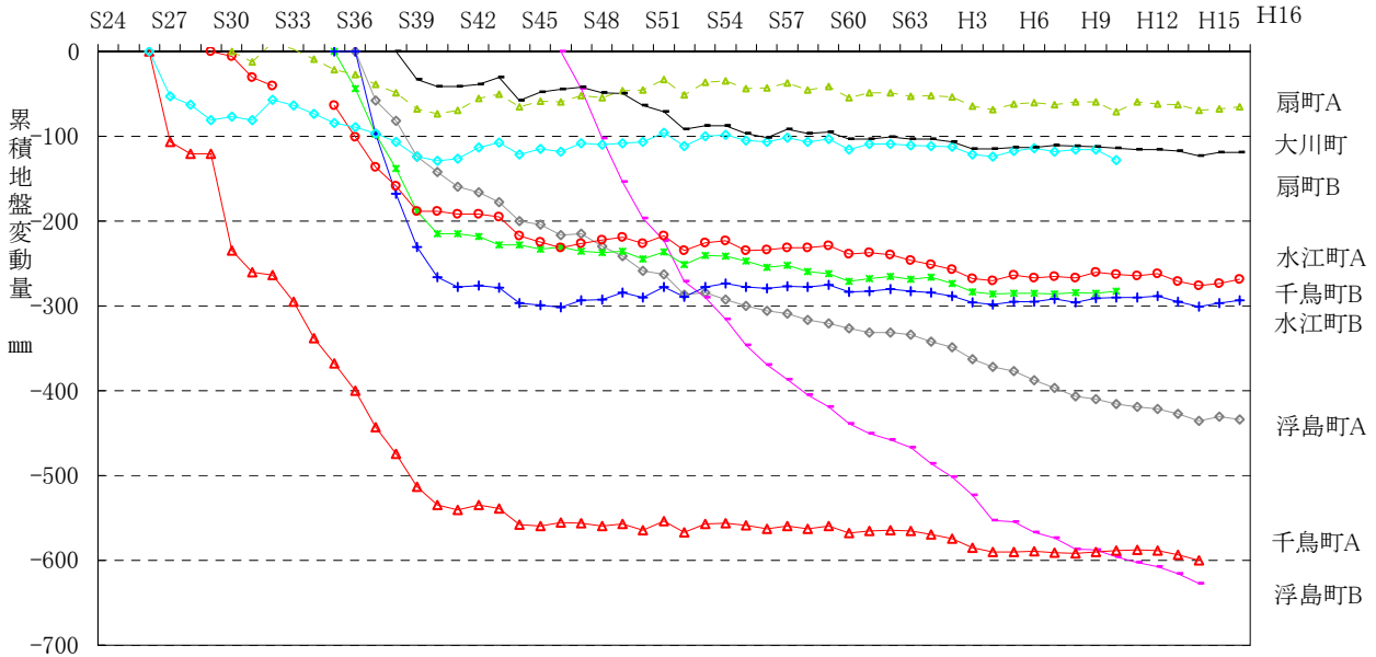
図9 主要水準点における累積地盤変動量の経年推移
