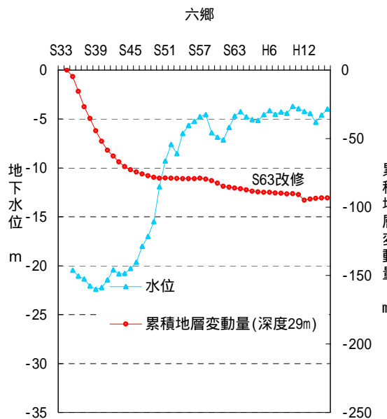
図 16 地下水位-累積地層変動量の経年推移
