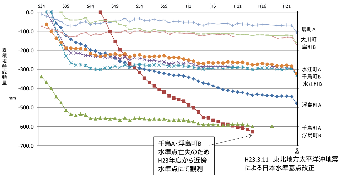
図 - 9 主要水準点における累積地盤変動量の経年推移 (~H23)
