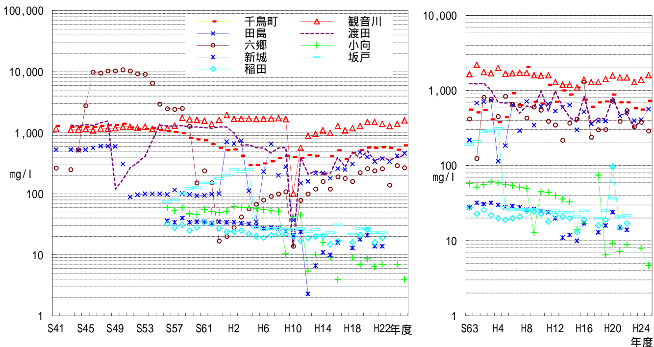
図 - 17 地下水塩化物イオン濃度の経年推移
