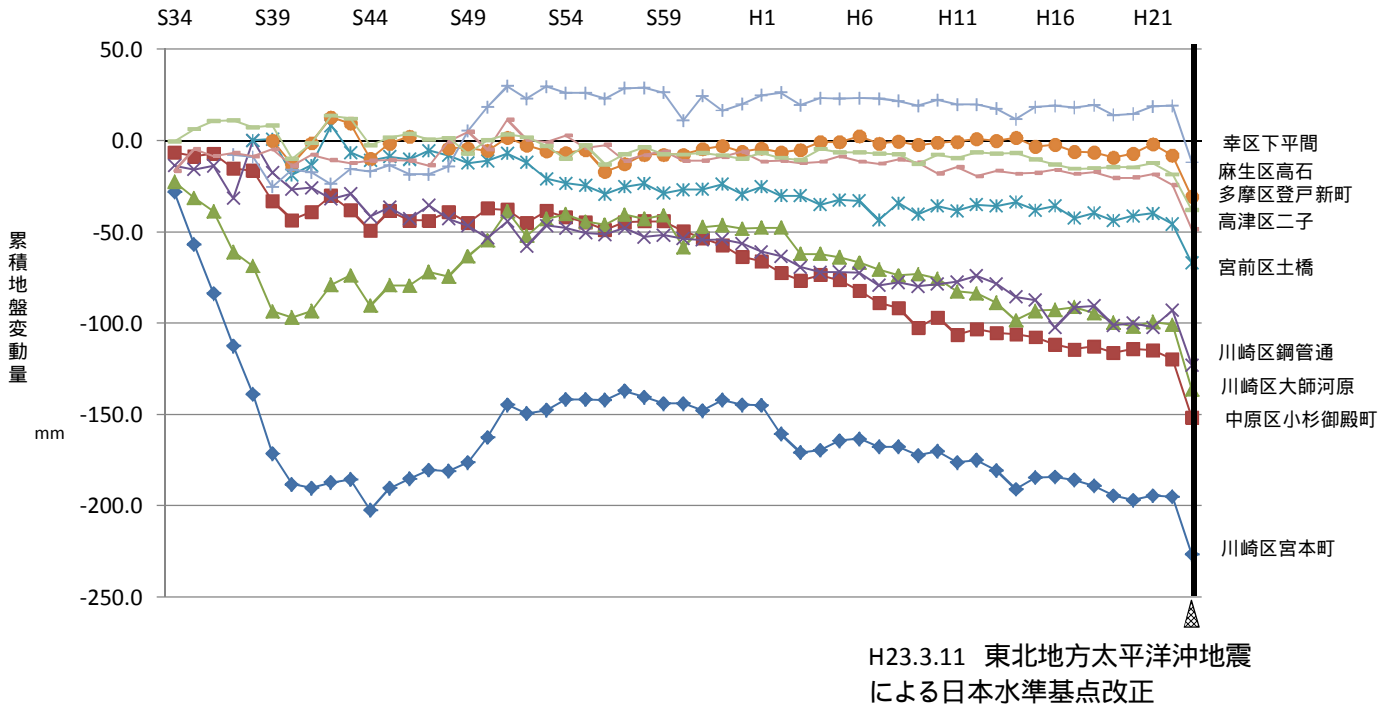
主要水準点における累積変動量の経年推移 (~H23)
