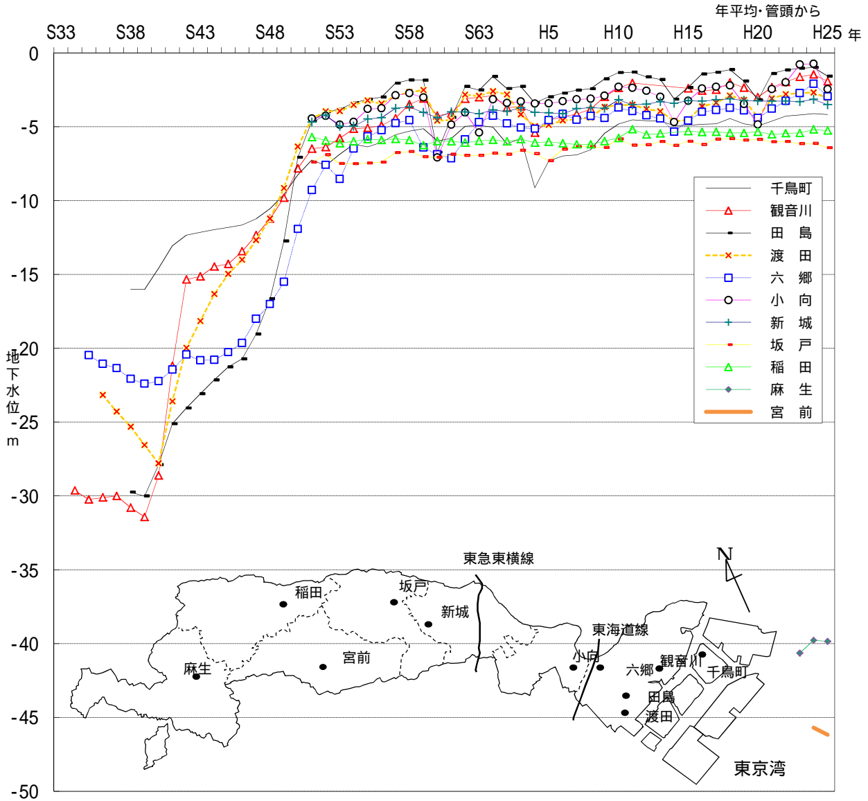
図 - 14 地下水位の経年推移
