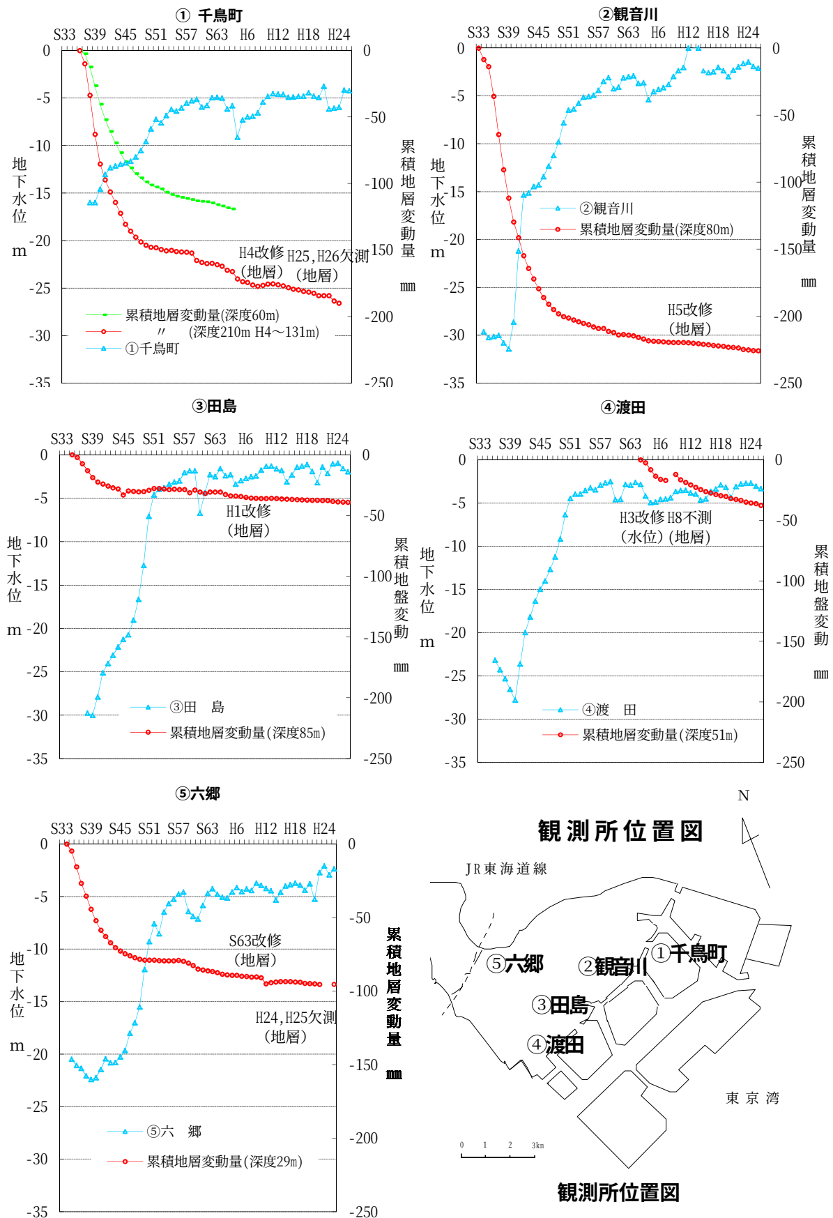
図V-16 地下水位-累積地層変動量の経年推移
