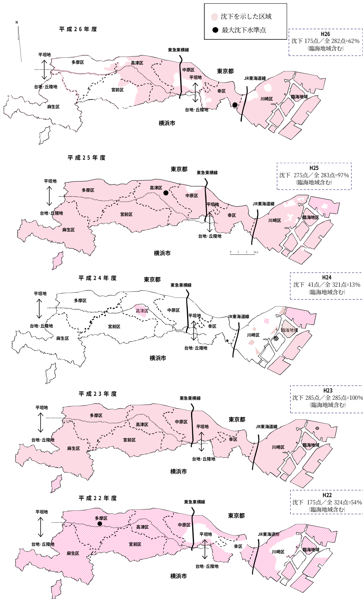
図V-5 地盤沈下区域の経年推移
