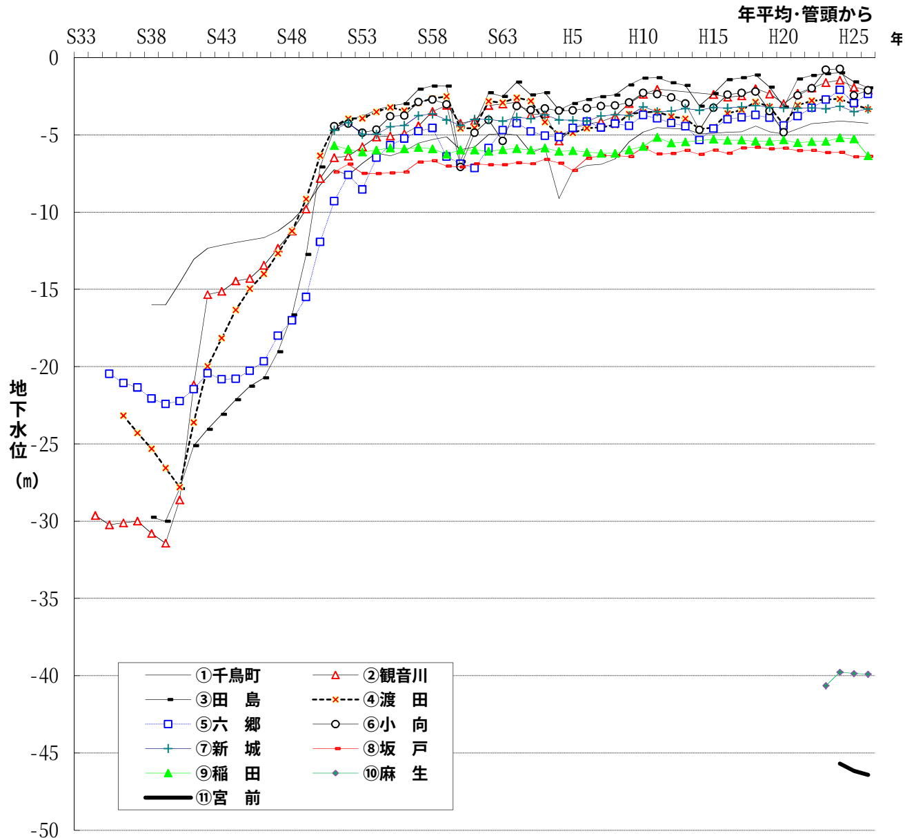
図V-14 地下水位の経年推移
