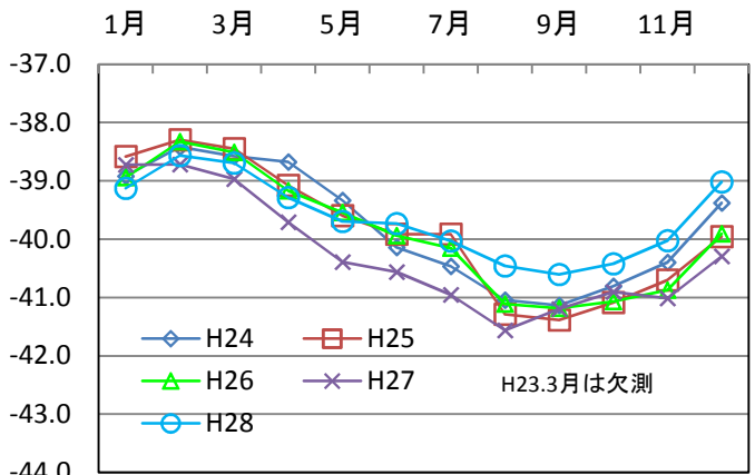
地下水水位[m] ⑩麻生
