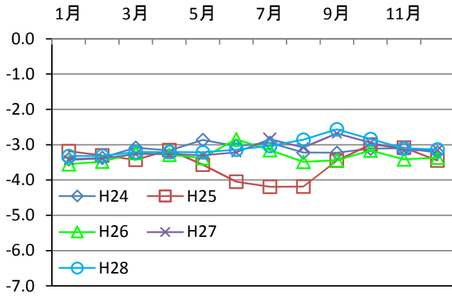
地下水水位[m] ⑦新城
