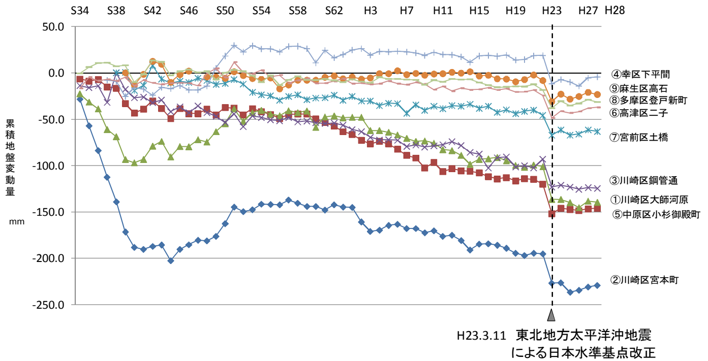
主要水準点における累積変動量の経年推移
