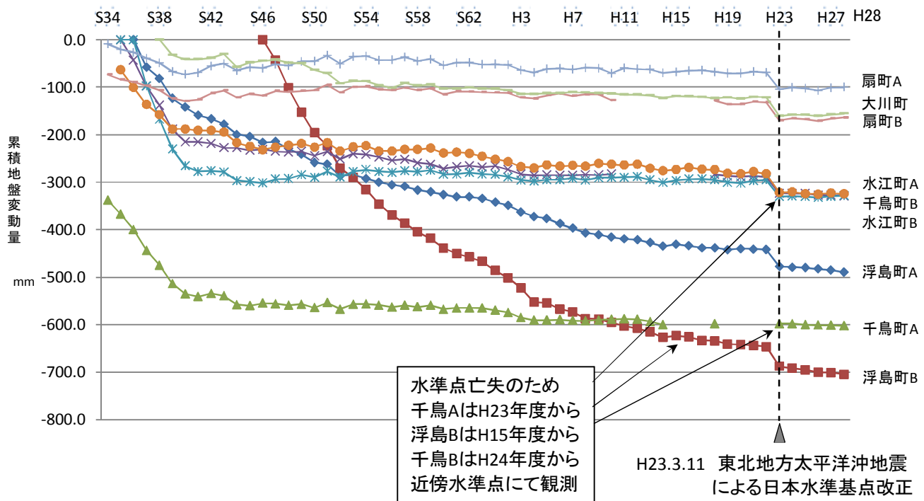
臨海地域における圧密沈下
