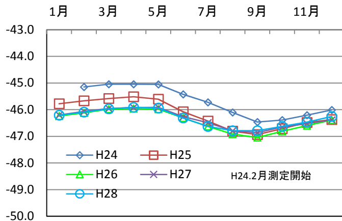
地下水水位[m] ⑪宮前
