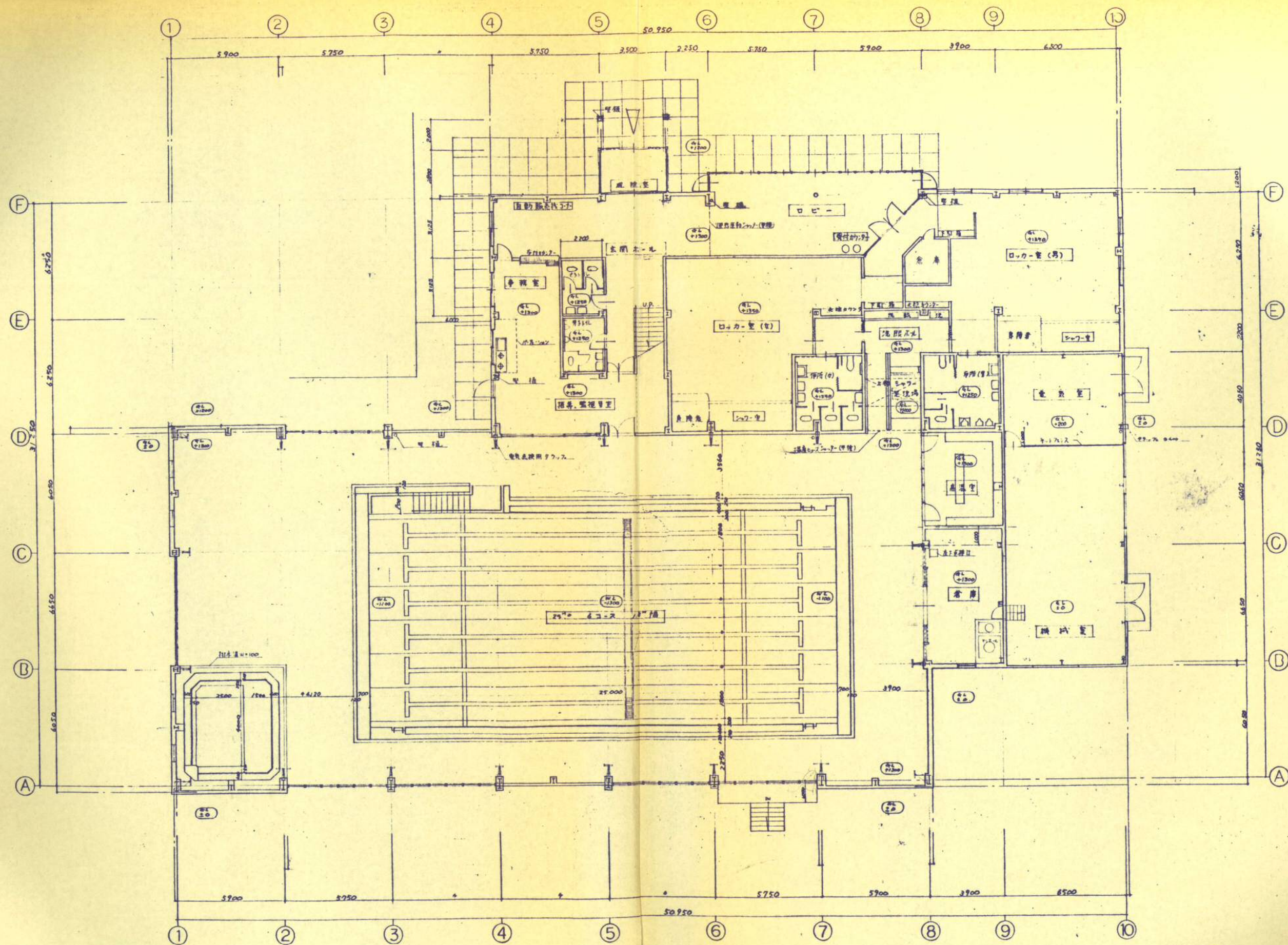
1F 1階平面図 S:1/200
