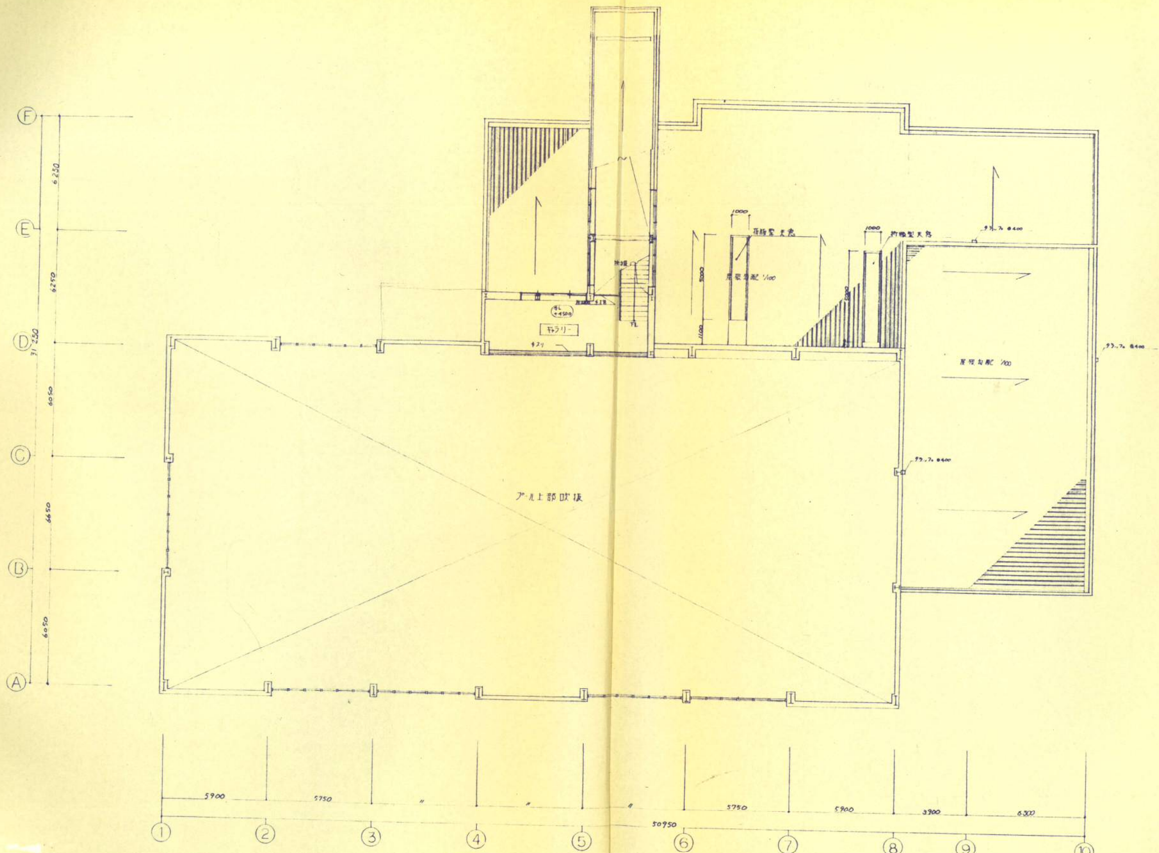
2階平面図及び屋根伏図 S: 1/100
