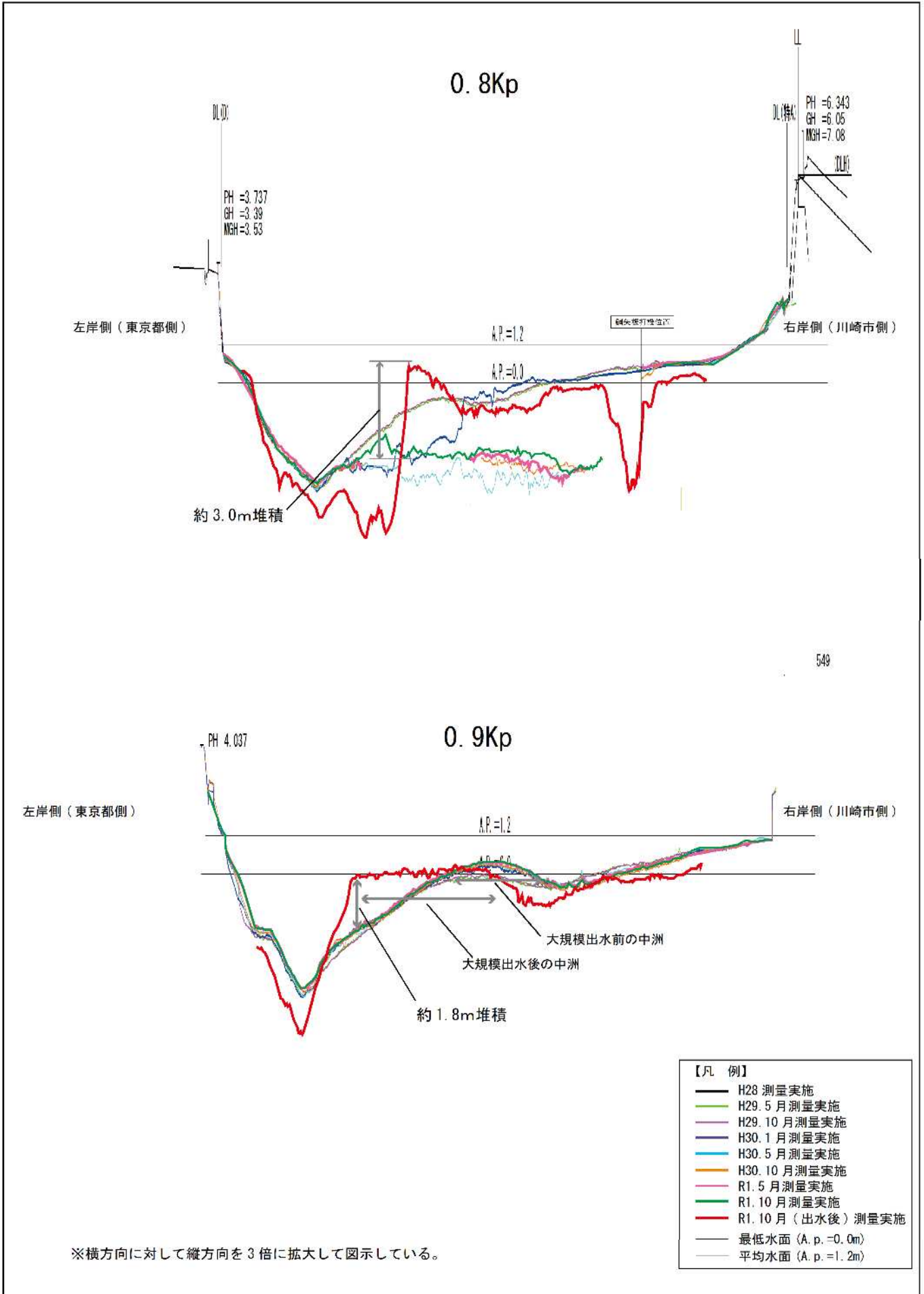
図 2.2(5) 河川横断面図(0.8kp ~ 0.9kp 地点)
