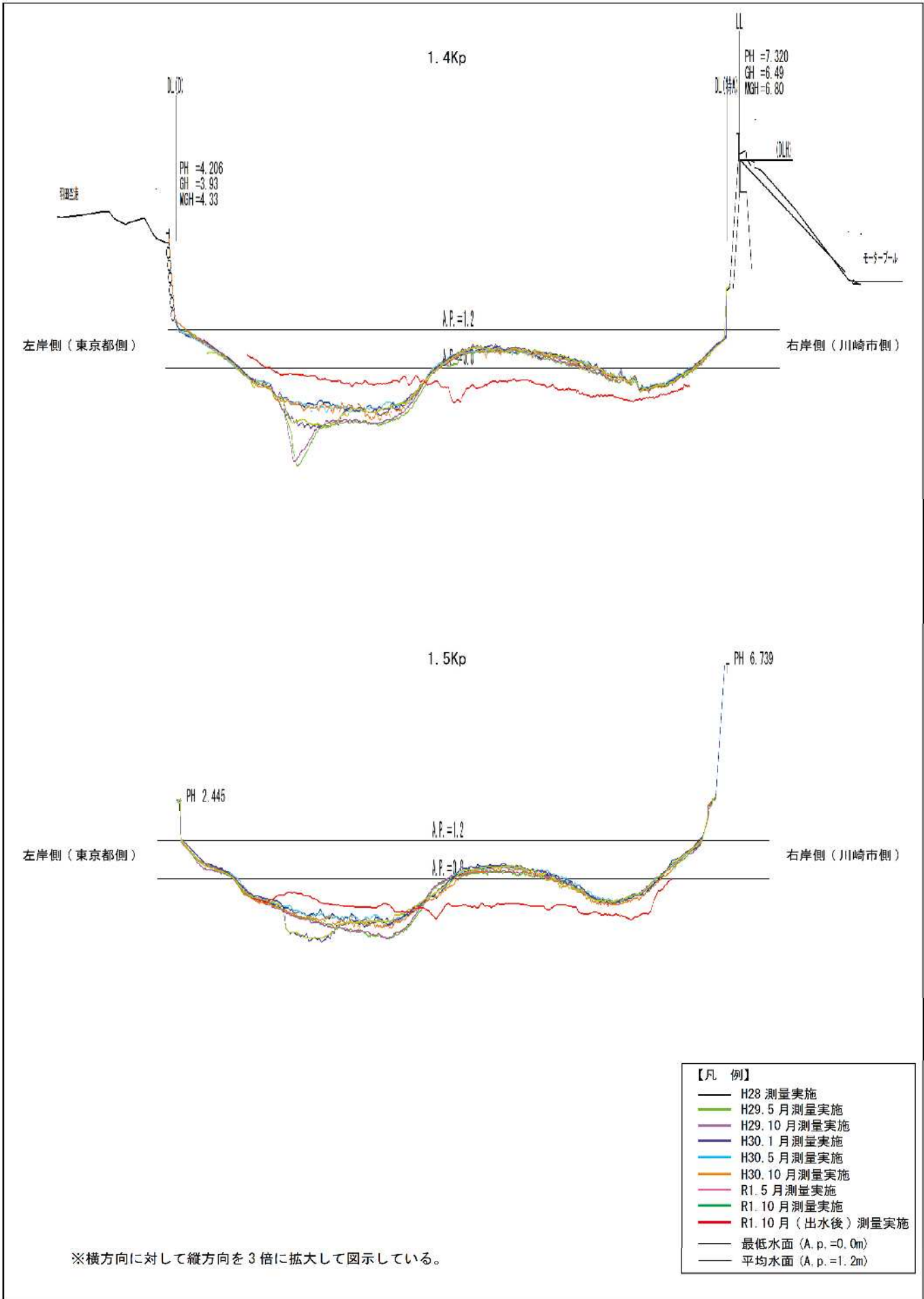
図 2.2(8) 河川横断面図(1.4kp ~ 1.5kp 地点)
