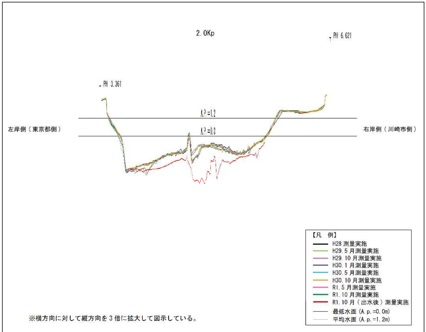
図 2.2(11) 河川横断面図(2.0kp 地点)
