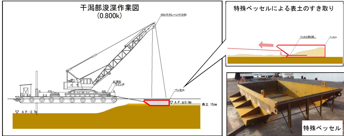
図 2.16 特殊ベッセルによる干潟部の表土すき取り方法
