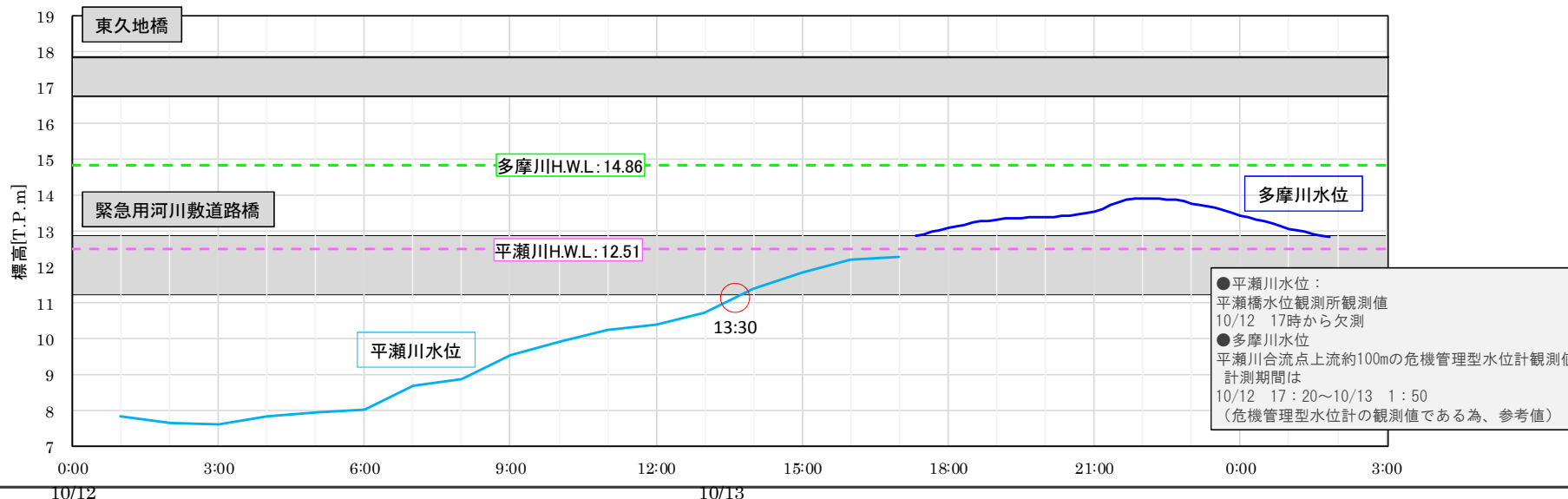
【平瀬川（多摩川合流部周辺）の水位と緊急用河川敷道路橋の高さ】
