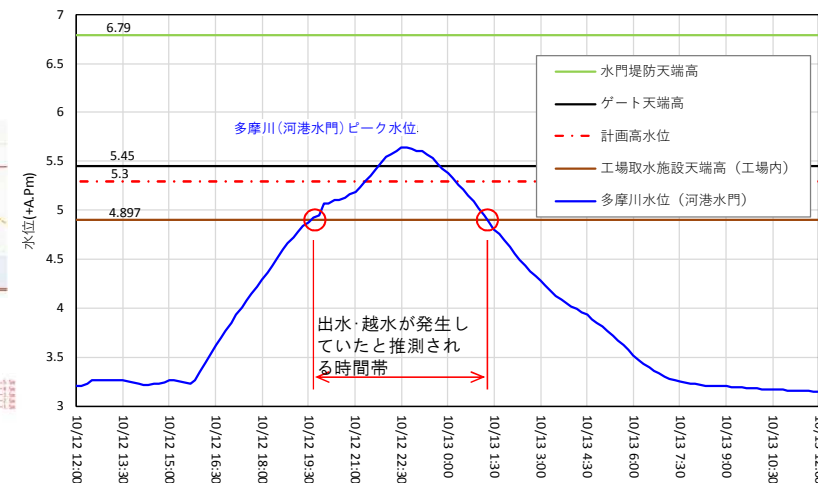
多摩川水位(河港水門)は、六郷橋下流水位観測所(約200m上流)の水位を縦断勾配をもとに河港水門の水位に換算した値である。(A. P.=T. P. - 1.134メートル)
