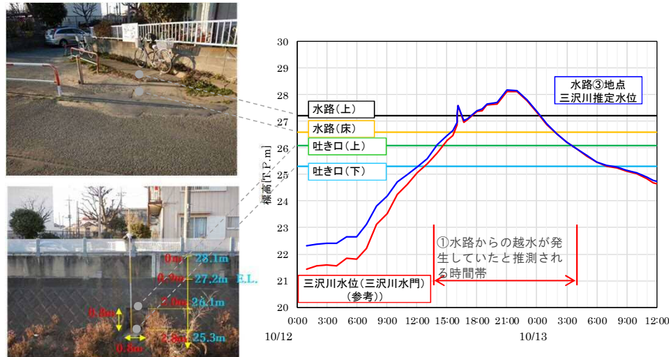
【吐き口部状況写真】
