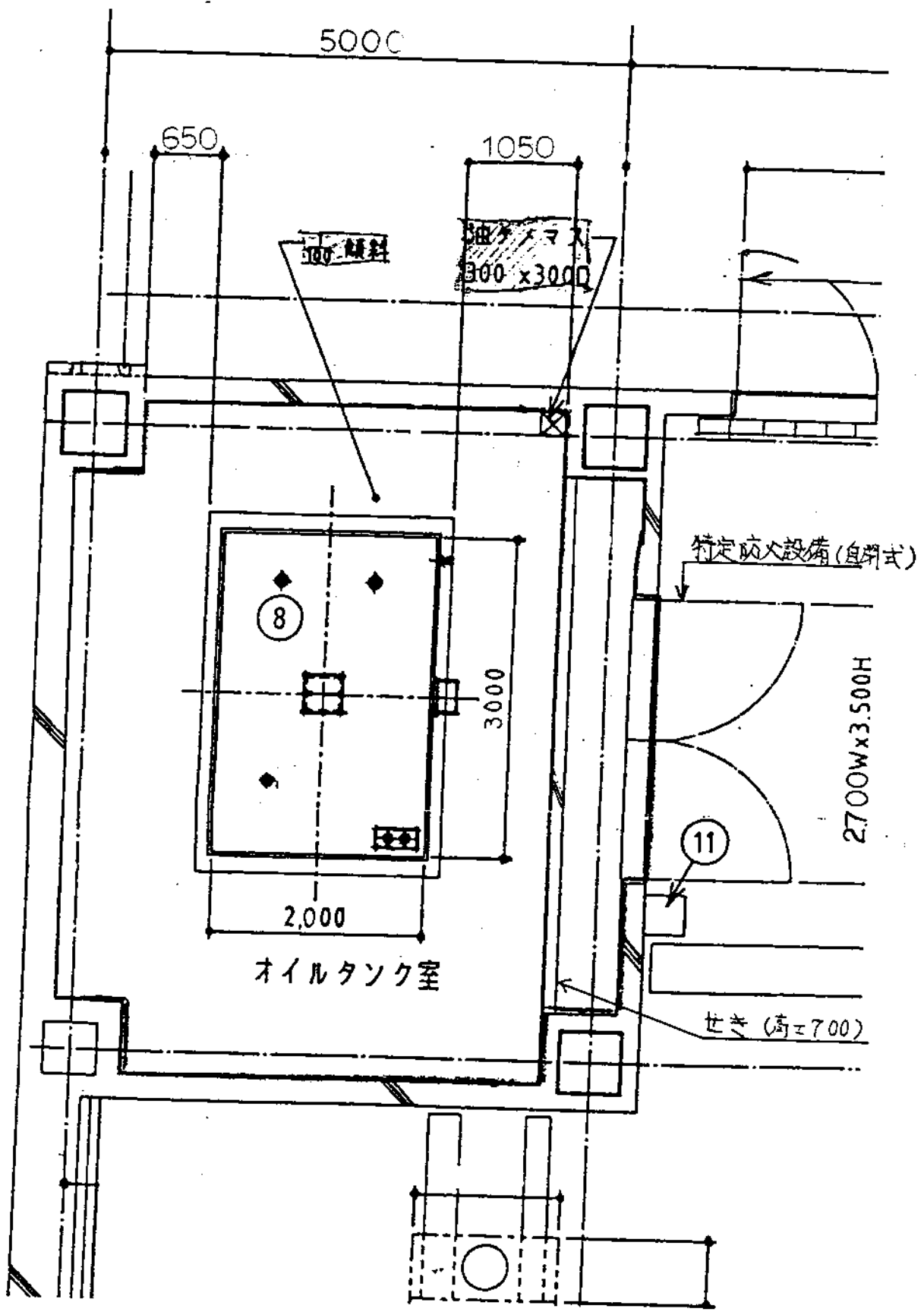
タンク専用室平面図
