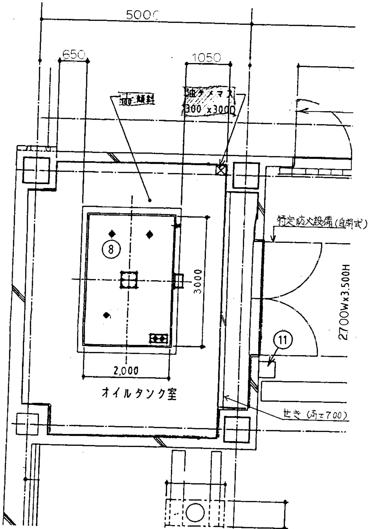
タンク専用室平面図 (囲い, タメマス詳細図)
