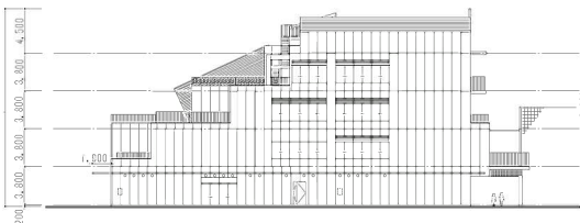
A: 西側立面図 (住宅地側)
