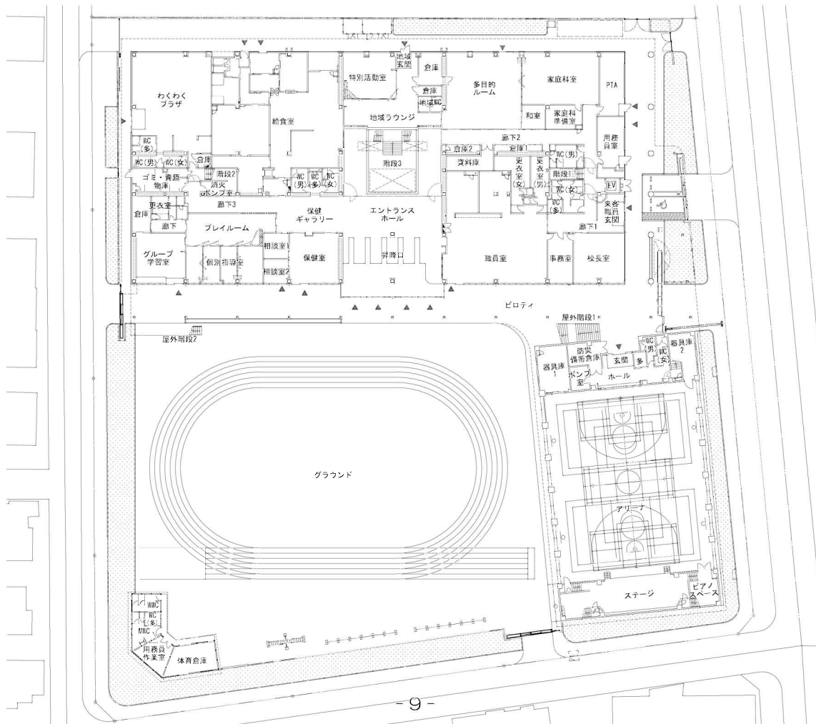
S=1/800 1階平面図
