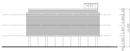
C: 南側立面図 (体育館)
