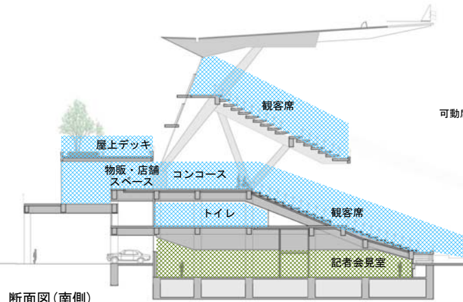
断面図(南側)
