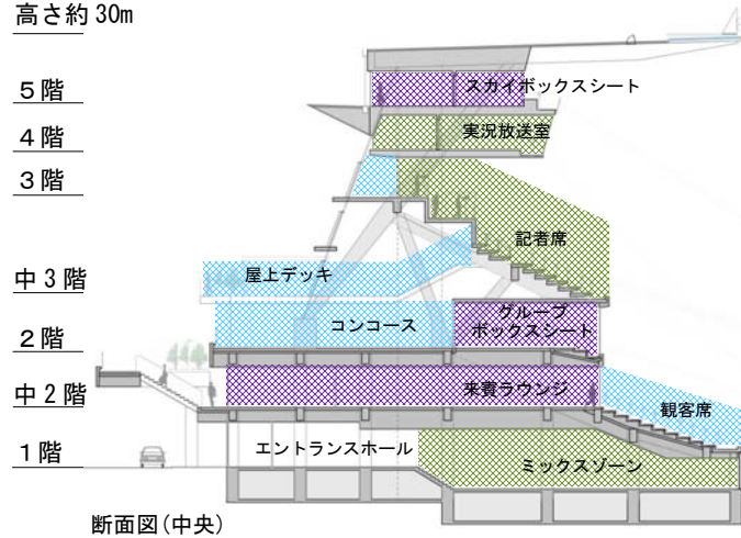
断面図(中央)
