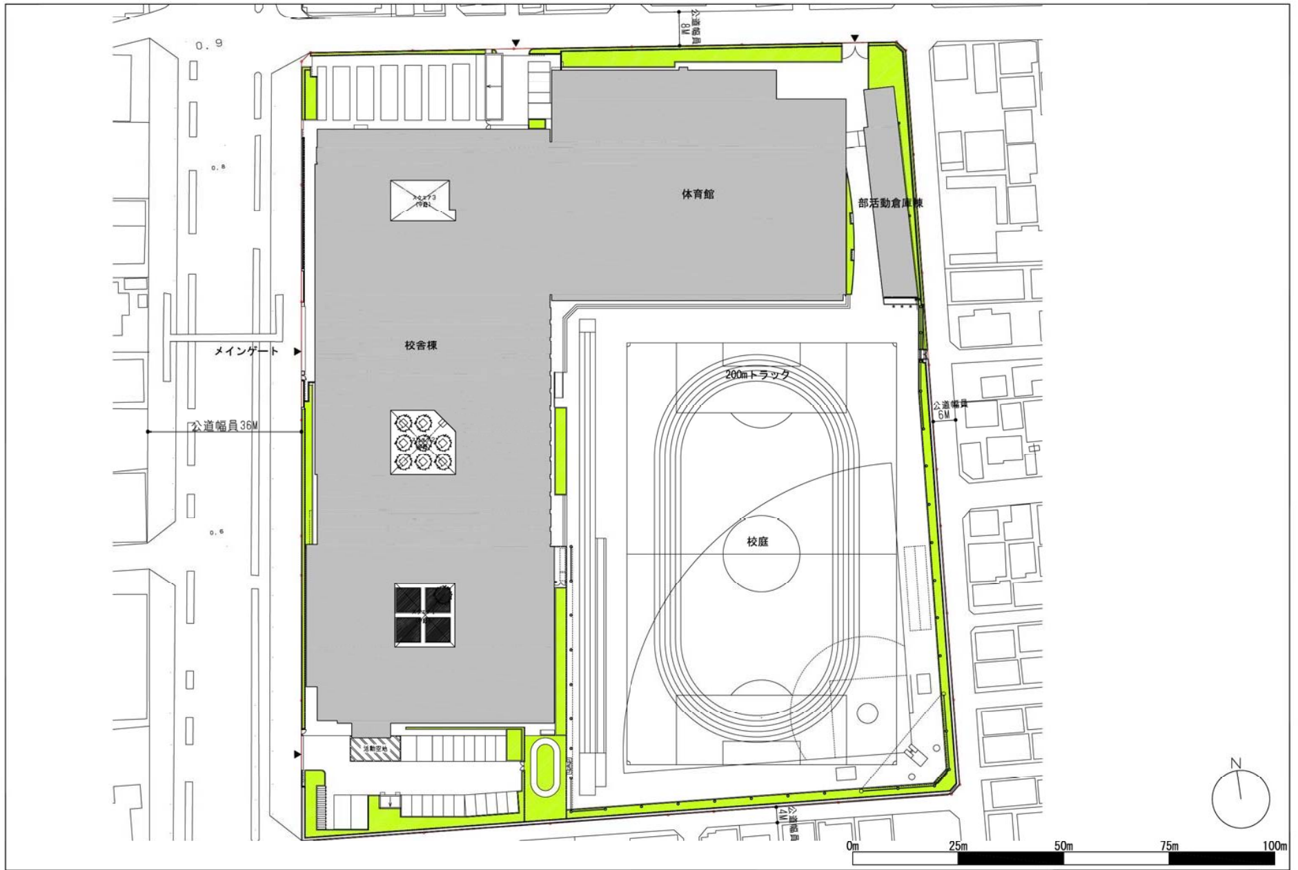
配置図 2
