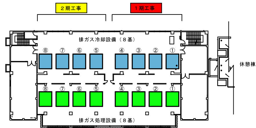
火葬棟 2階平面図
