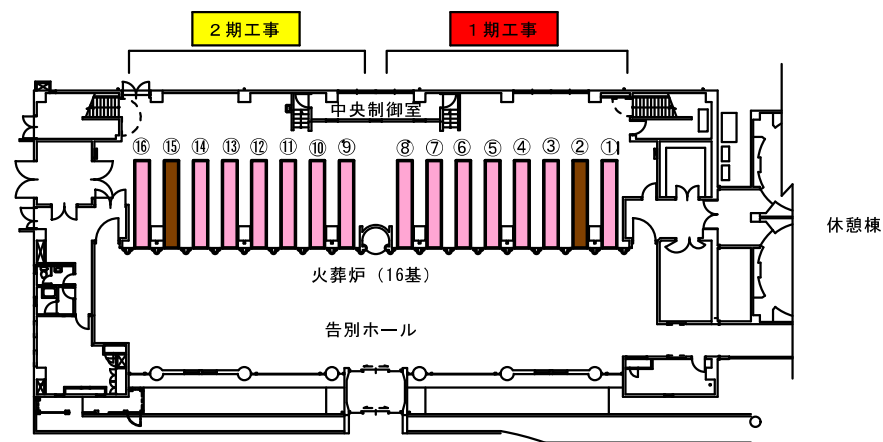
火葬棟 1階平面図
