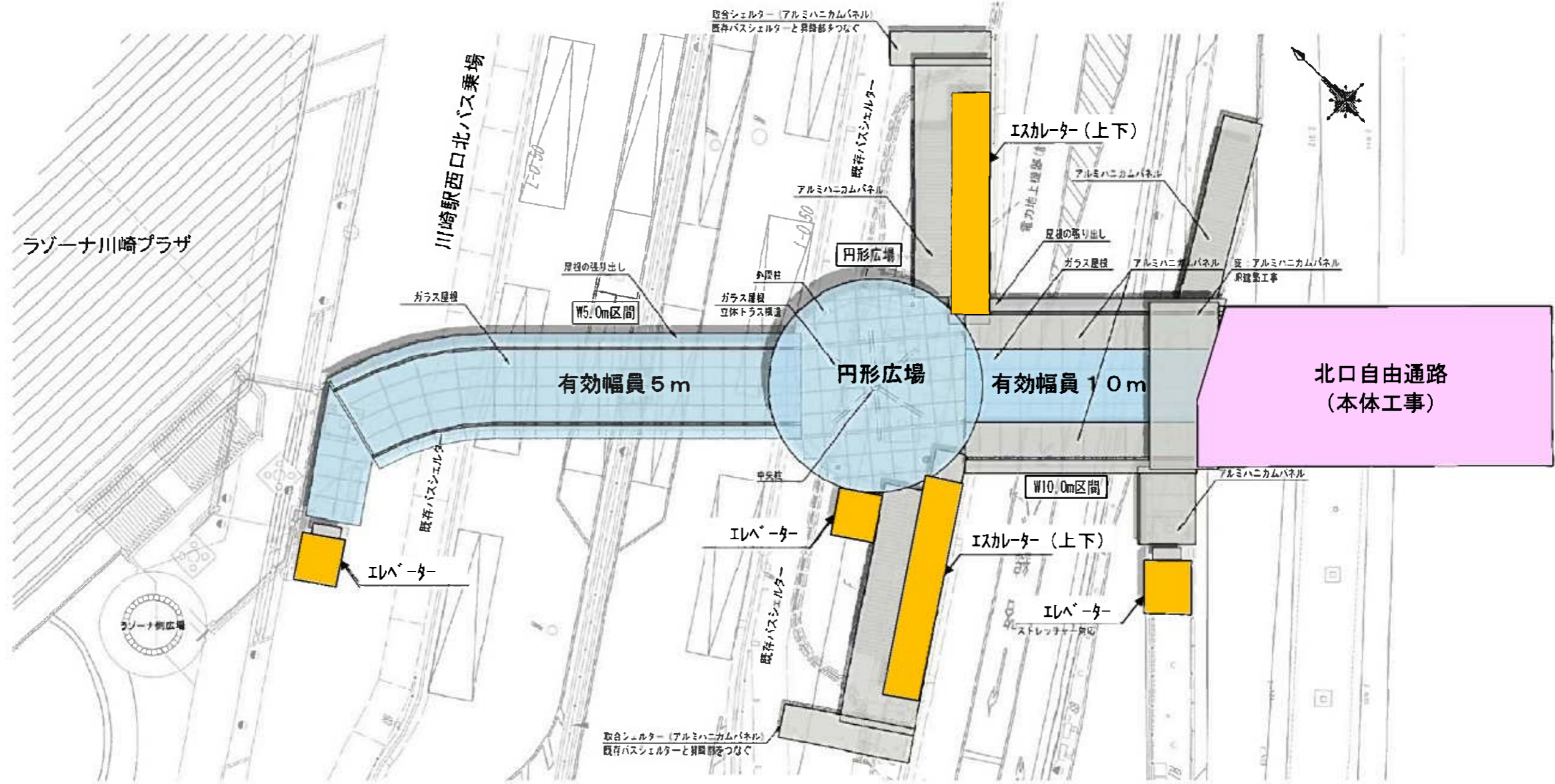
平面図
