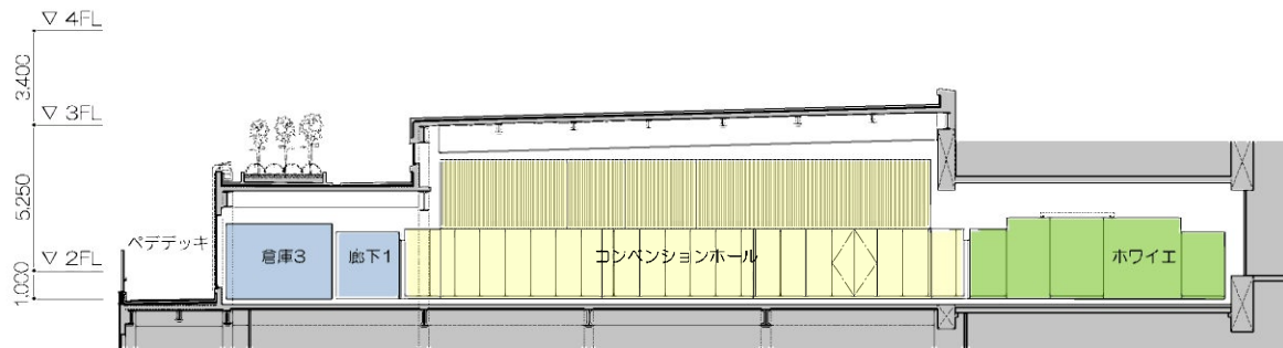
断面図-2
