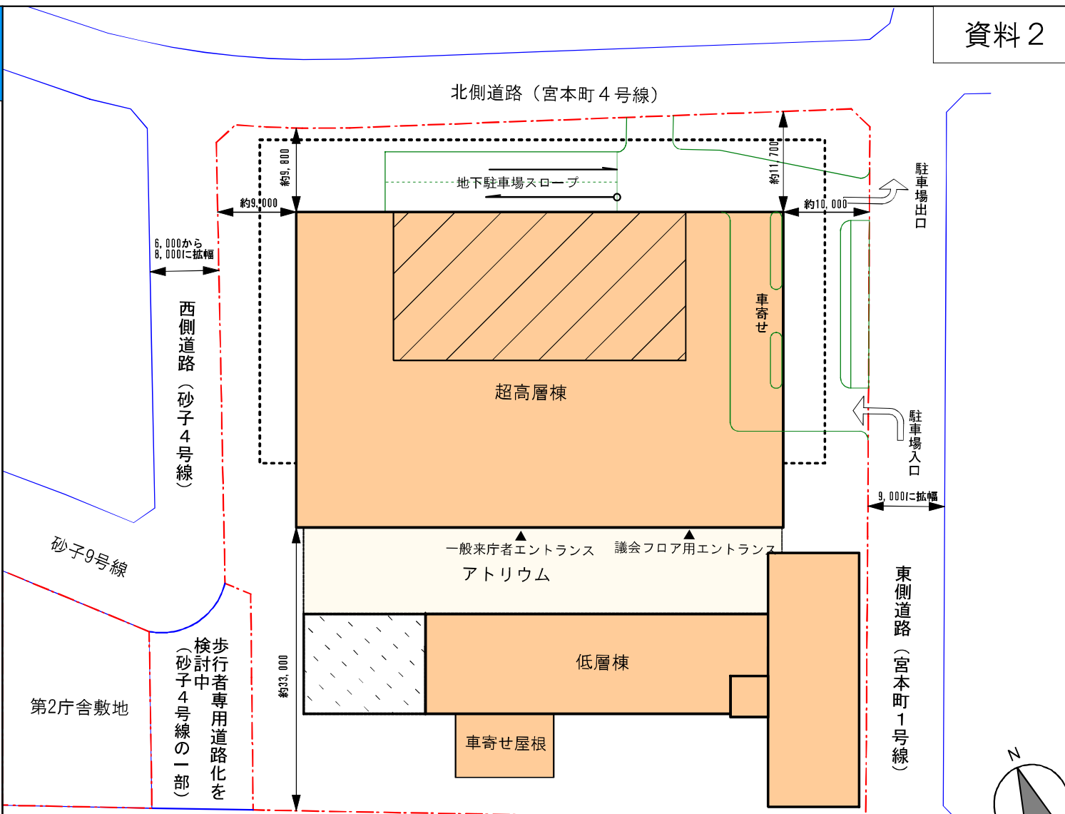
配置図 S=1:600
