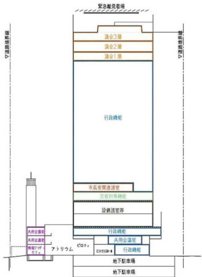
南北断面図
