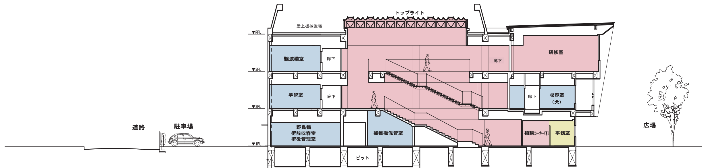
A-A' 断面図
