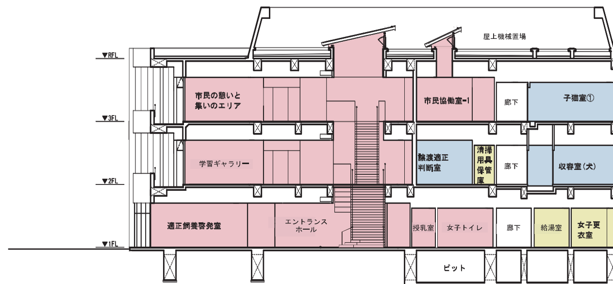
B-B' 断面図
