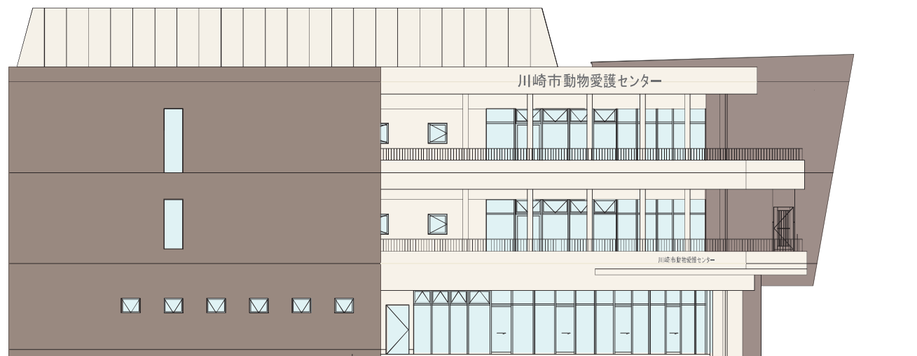
西側立面図
