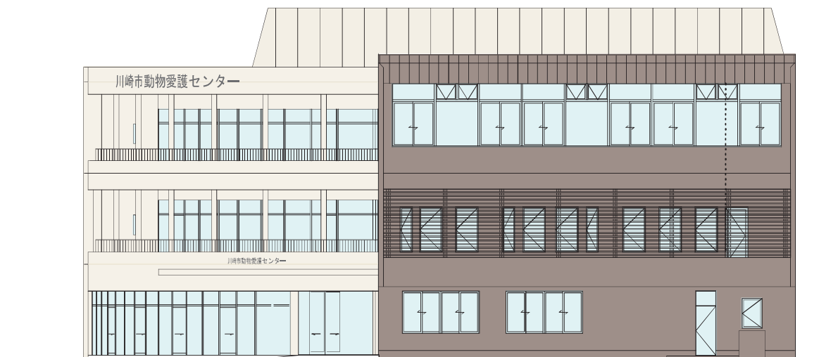
南側立面図
