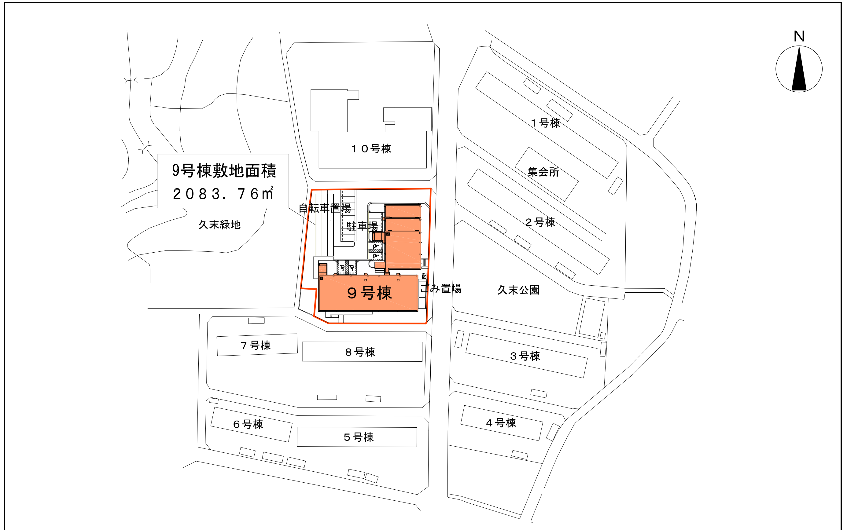
全体配置図 S=1/800
