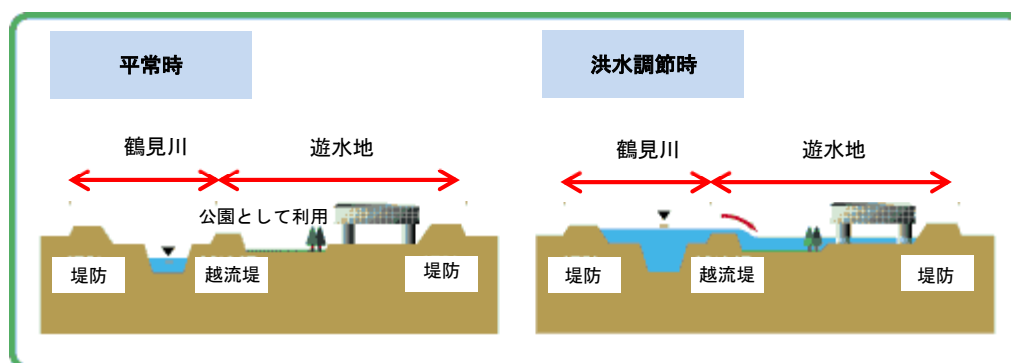
鶴見川多目的遊水地の概略図（横浜市HPより）
