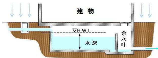
地下貯留槽概要図
