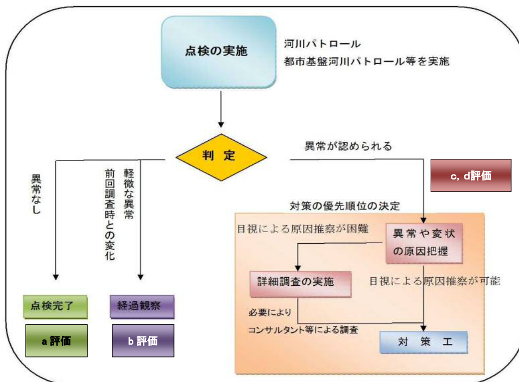
図 5.3 点検フロー
