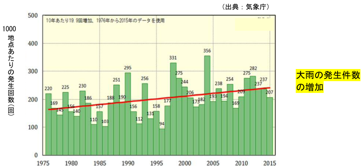
図 1.5 1 時間降水量 50mm 異常の年間発生回数 (1976 年～)
