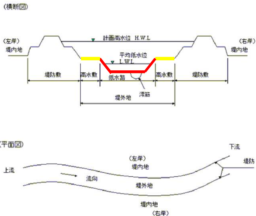
図 10.1 河川一般図
