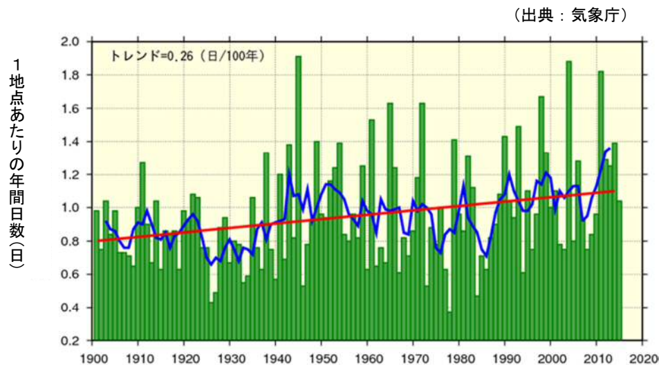
図 1.6 日降水量 100mm 以上の年間日数(1900 年～)
