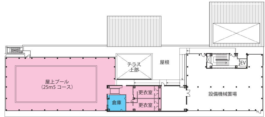
5階平面図 S=1/600
