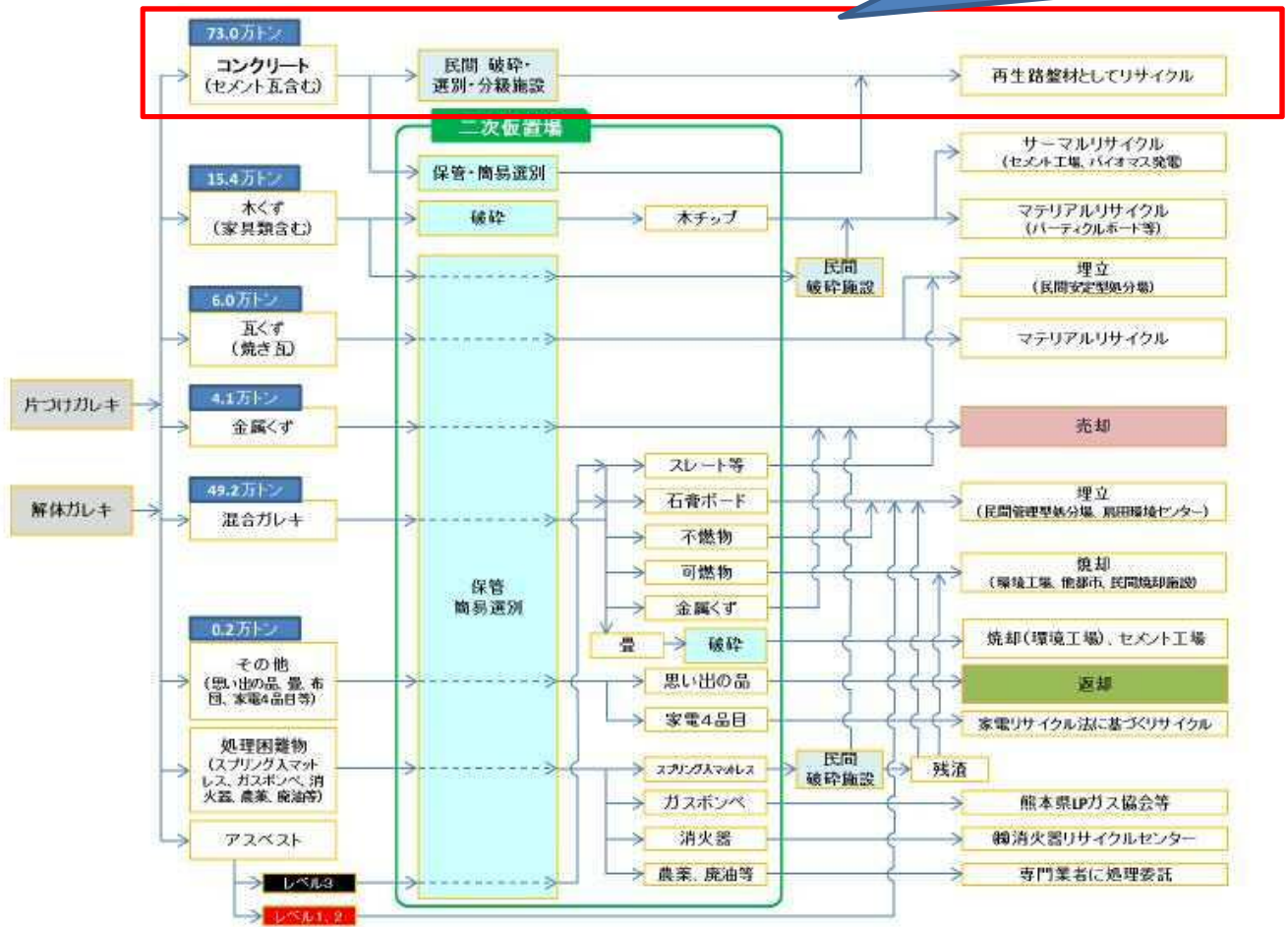
図3-8 熊本地震に伴う災害廃棄物の処理フロー (「平成28年4月熊本地震に係る熊本市災害廃棄物処理実行計画第3版」を編集)
