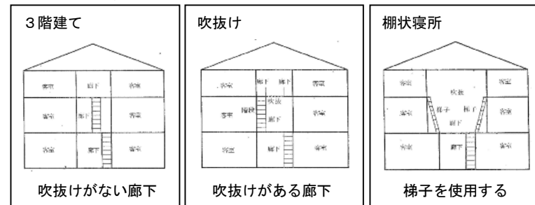
簡易宿所の代表的なパターン（木造で3層を有するもの）
