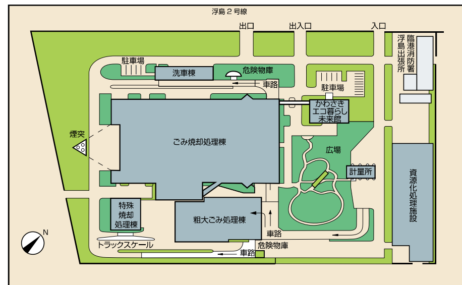
施設配置図
