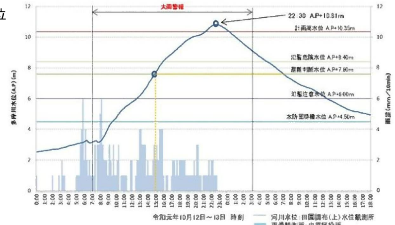
令和元年10月12日~13日 時刻 河川水位：田園調布(上)水位観測所 雨量観測所：中原区役所 山王排水樋管地域の降雨量と田園調布(上)の多摩川水位
