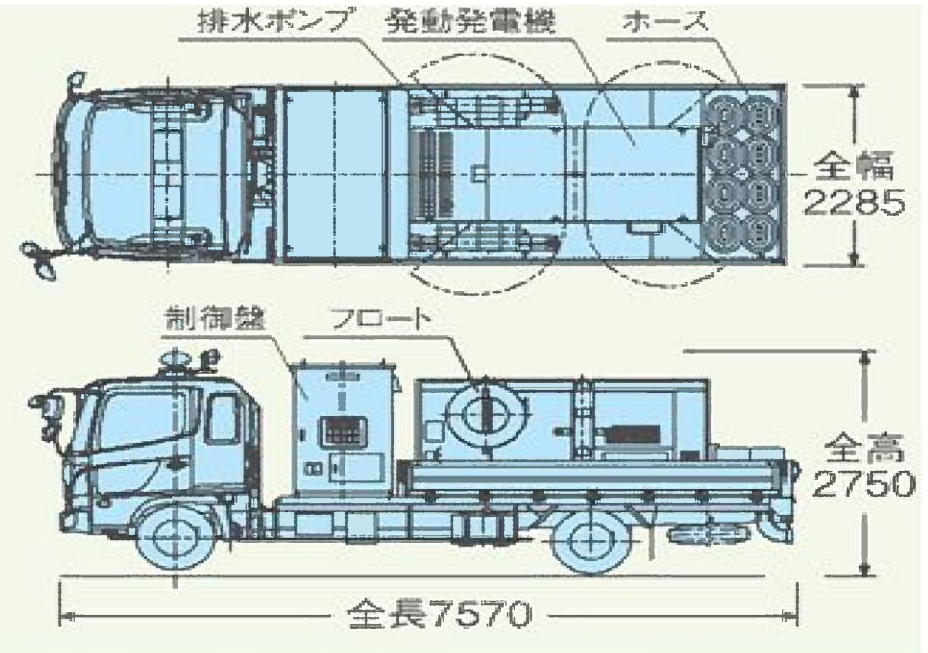
外形図
