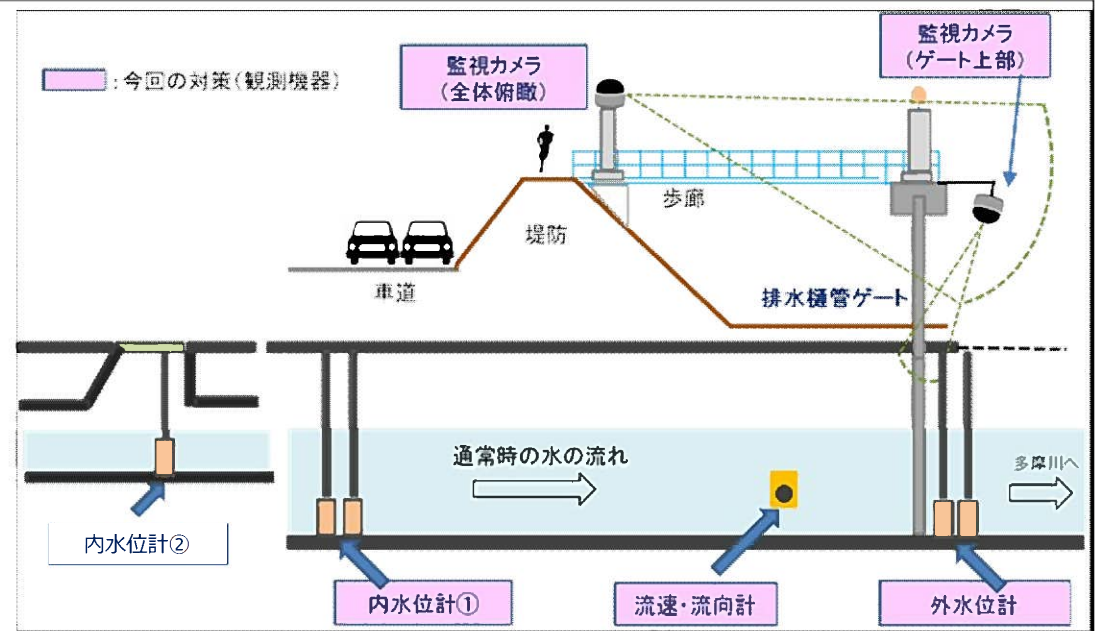
観測機器の設置イメージ
