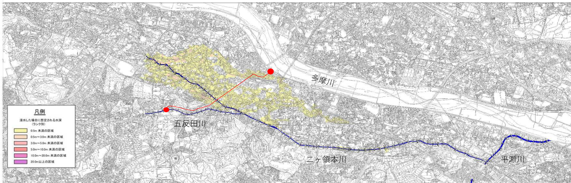
90mm降雨時の浸水想定面積 (156ha) [30年に1回程度]
