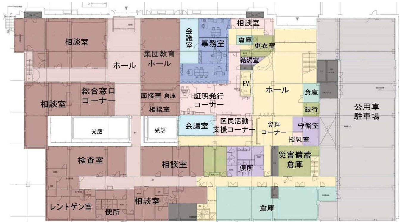
■1階平面図
