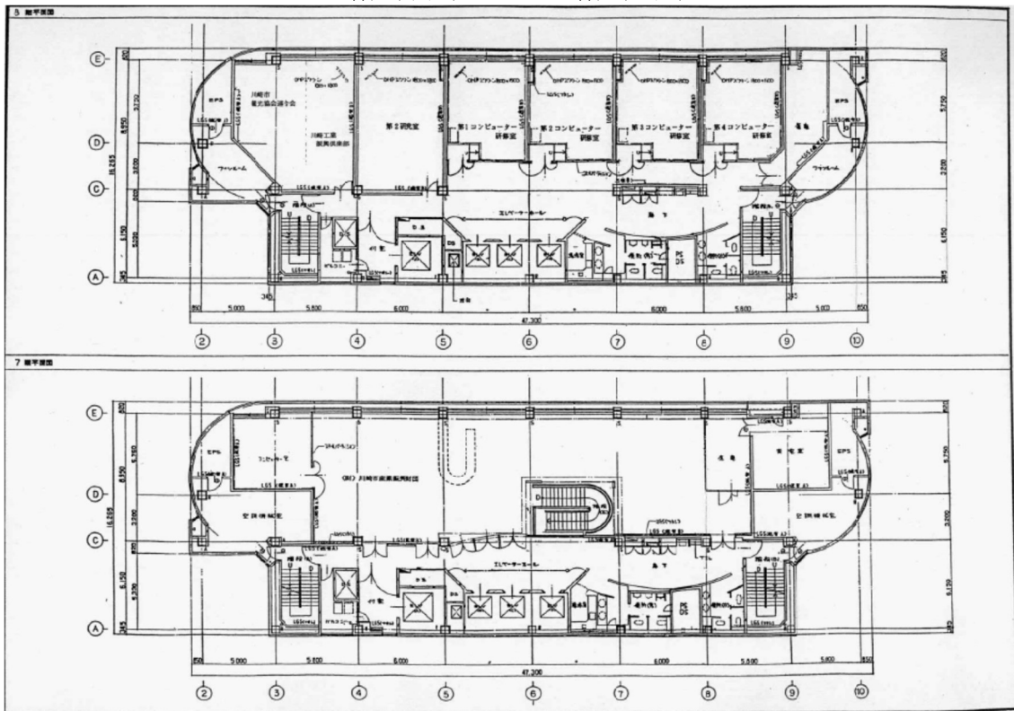
7階（下図） および8階（上図）
