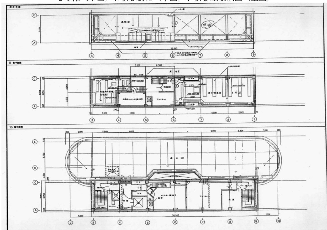
1 3 階 (下図) および R 階 (中図) および屋根伏図 (上図)
