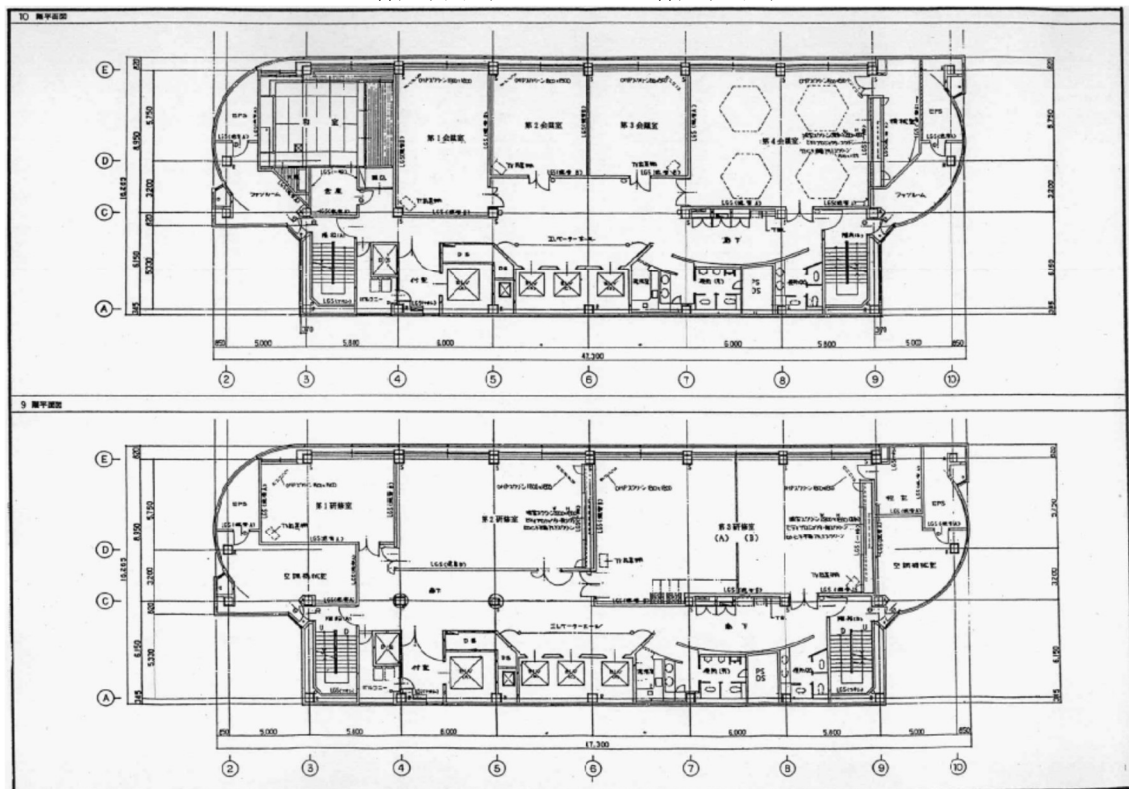
9階（下図） および10階（上図）
