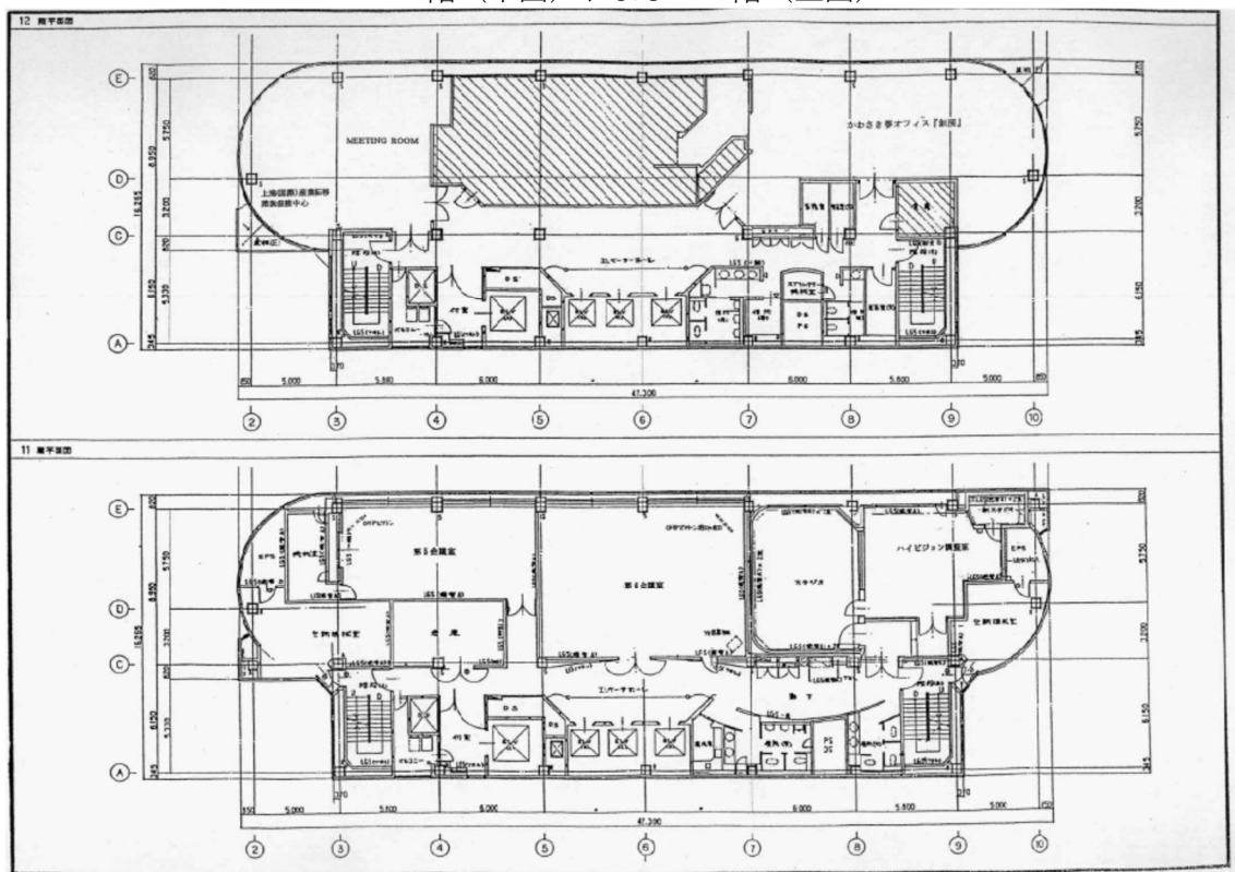
1 1 階 (下図) および 1 2 階 (上図)
