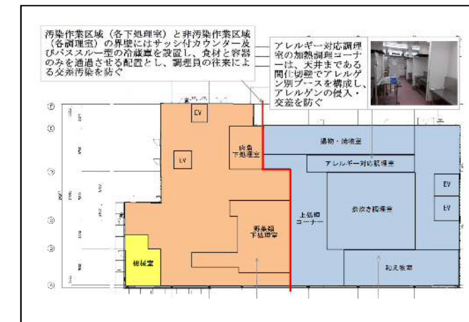
3階 平面図
