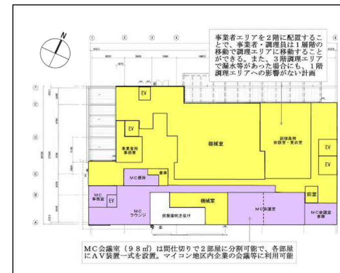
2階 平面図
