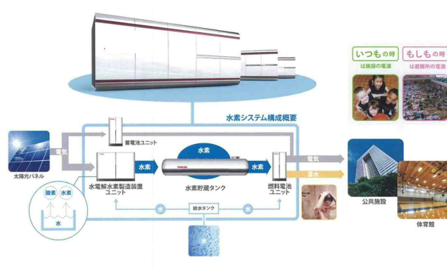
再生可能エネルギー由来の水素を用いた 自立型エネルギー供給システム
