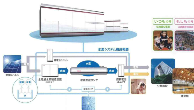
再生可能エネルギー由来の水素を用いた 自立型エネルギー供給システム
