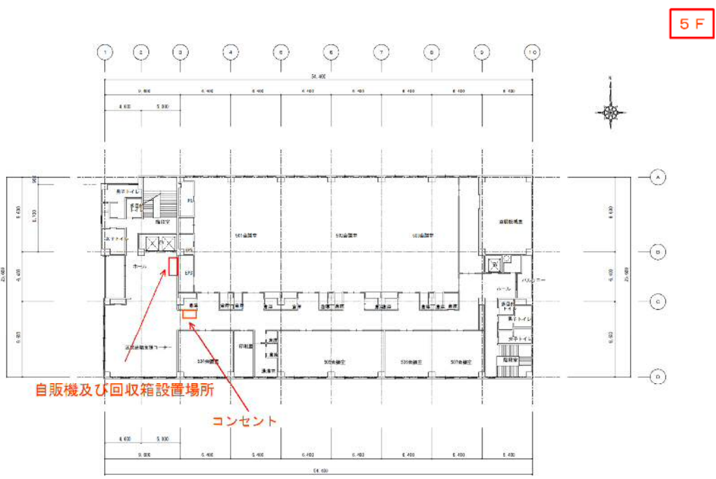
中原区役所 5階平面図 S-1/200
