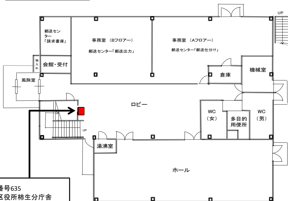
1階平面図
