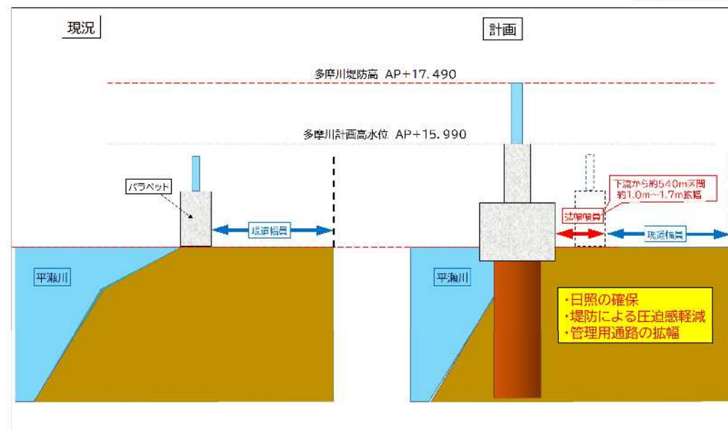
堤防イメージ図
