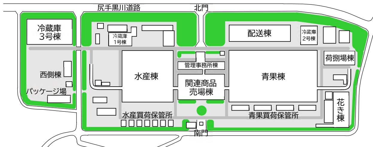
施設配置図
