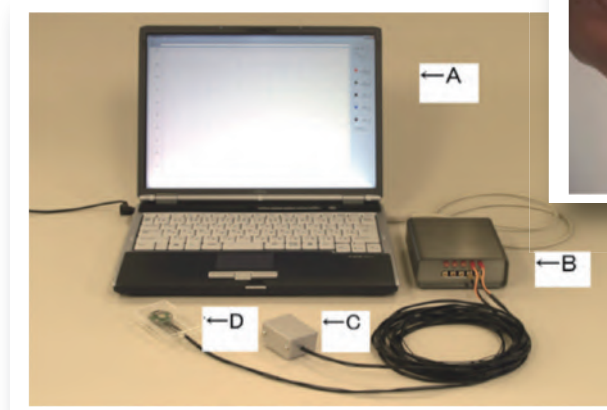
雰囲気分析装置の構成
