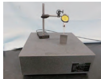
石定盤でも使える 真空吸着スタンド
