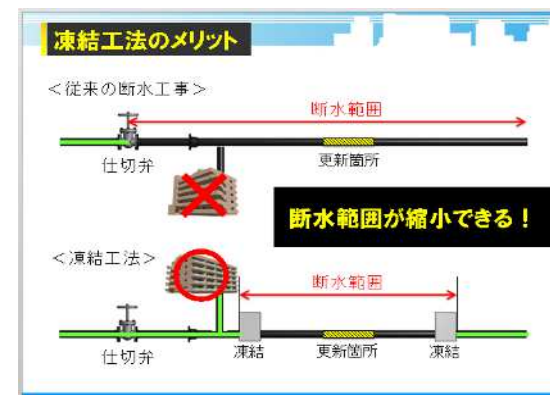
凍結工法のメリット
