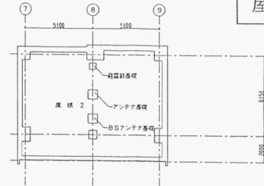
屋根伏図
