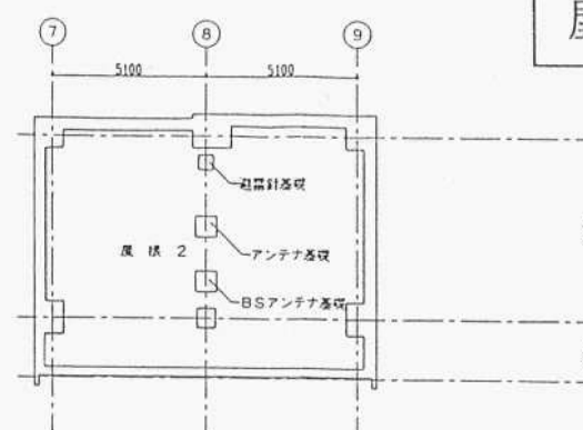
屋根伏図
