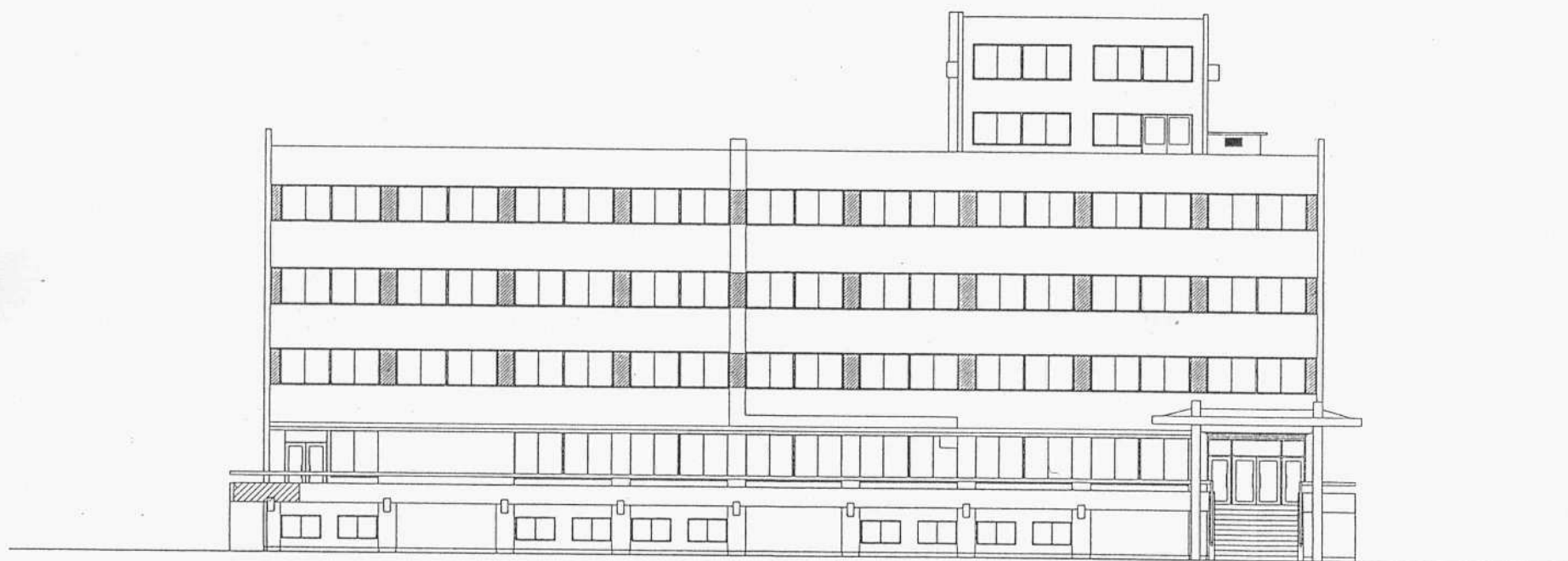
南側立面図
