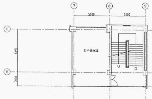
PH2階平面図
