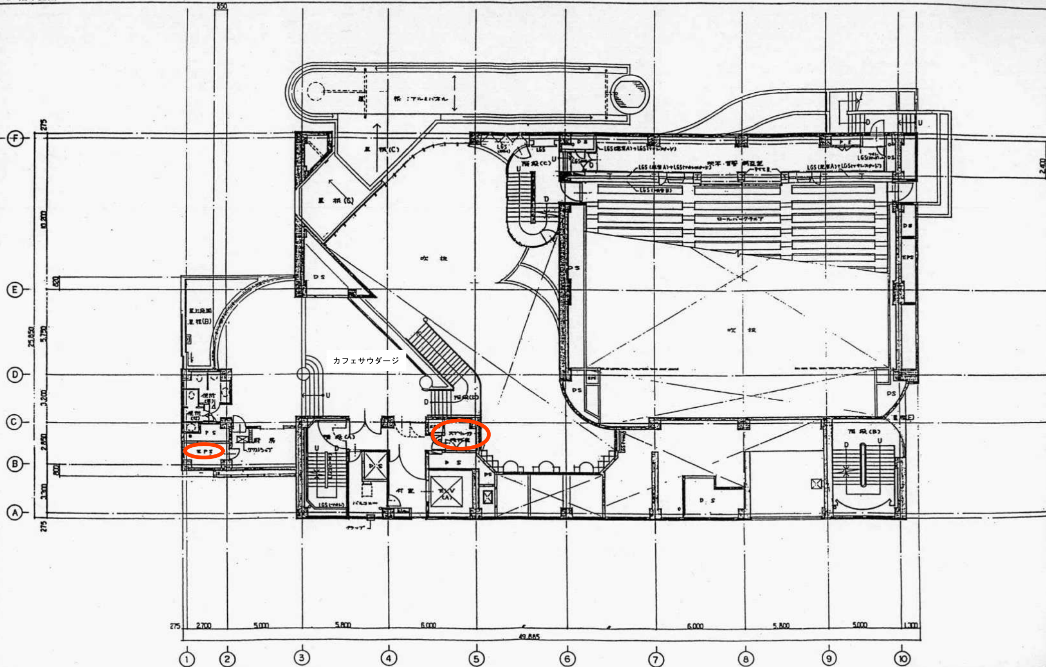
2 階平面図
