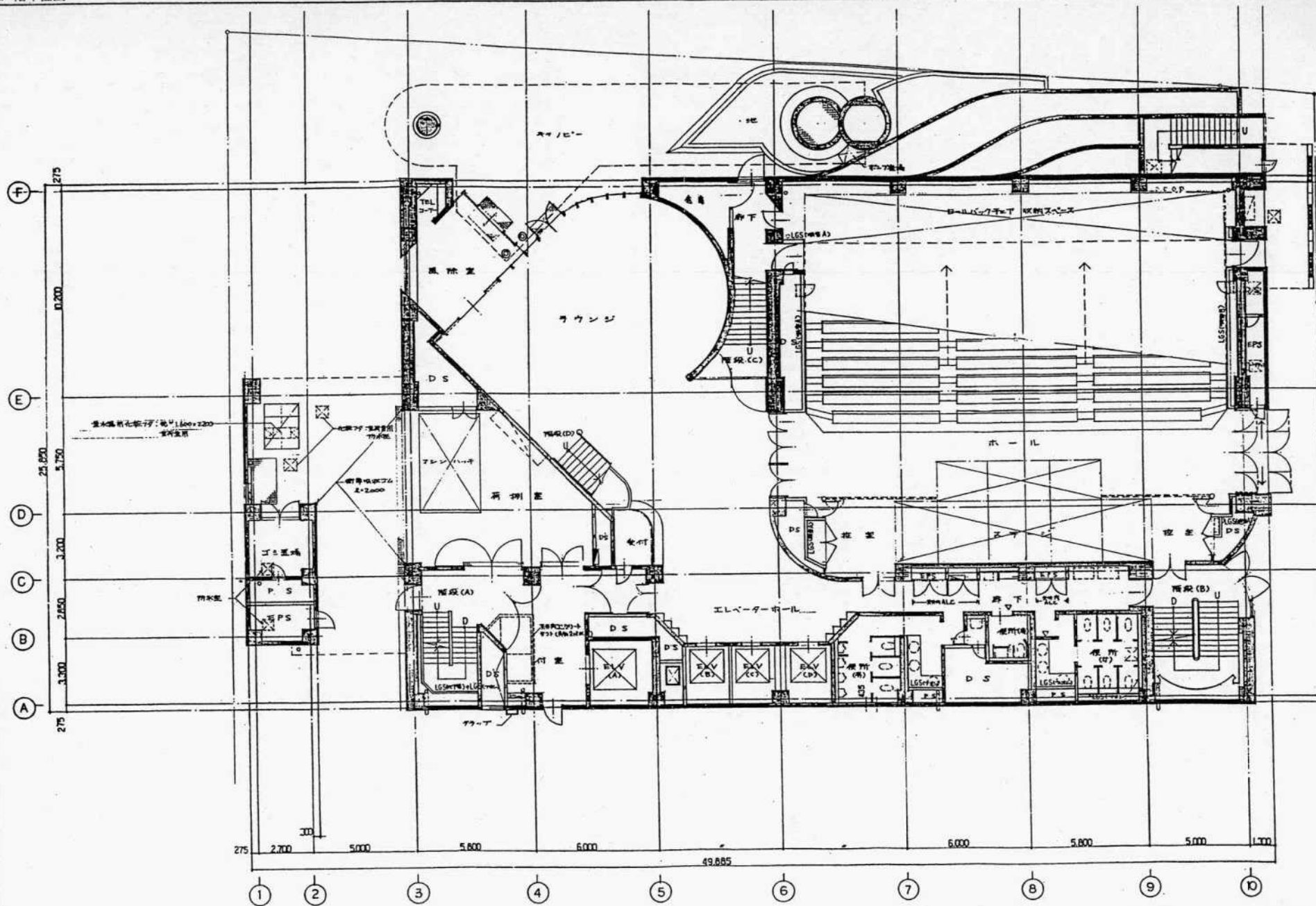
1 階平面図
