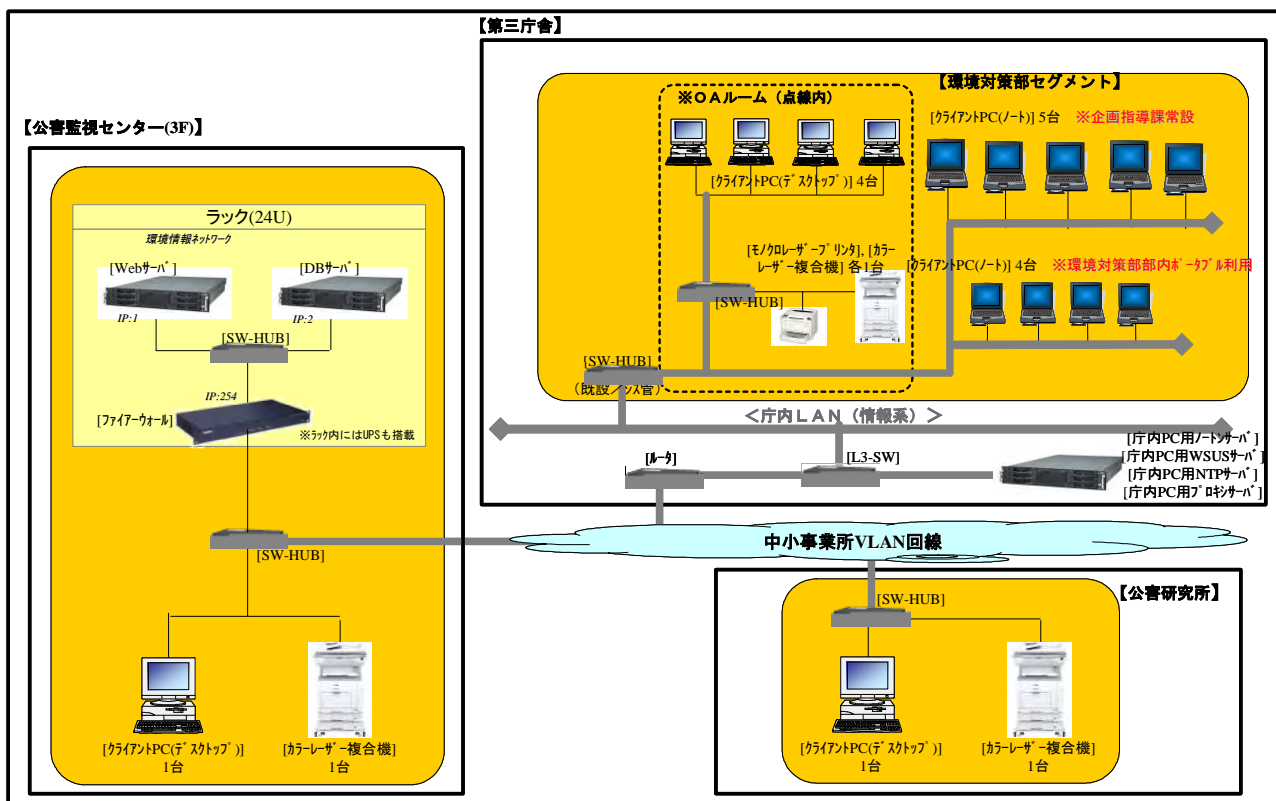
環境情報システムの構成概要
